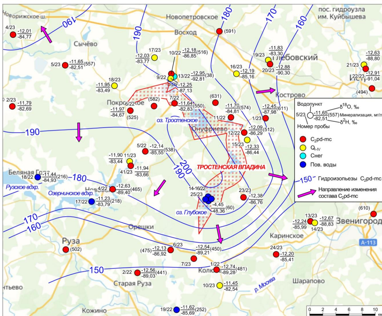
Рис. 1. Схема отбора проб природных вод с результатами опробования
