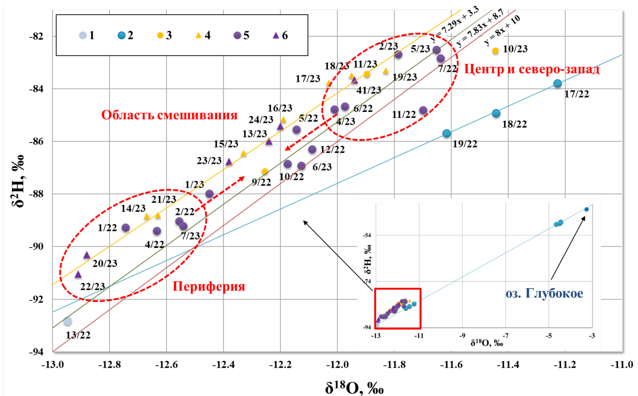
Рис. 2. График зависимости \delta^2\text{H} от \delta^{18}\text{O} в природных водах района исследования [14]: 1 – снег; 2 – поверхностные воды; 3 – четвертичный водоносный комплекс, опробованный в марте 2022 и 2023 гг.; 4 – четвертичный водоносный комплекс, опробованный в июне 2023 г.; 5 – подольско-мячковский водоносный комплекс, опробованный в марте 2022 и 2023 гг.; 6 – подольско-мячковский водоносный комплекс, опробованный в июне 2023 г.
