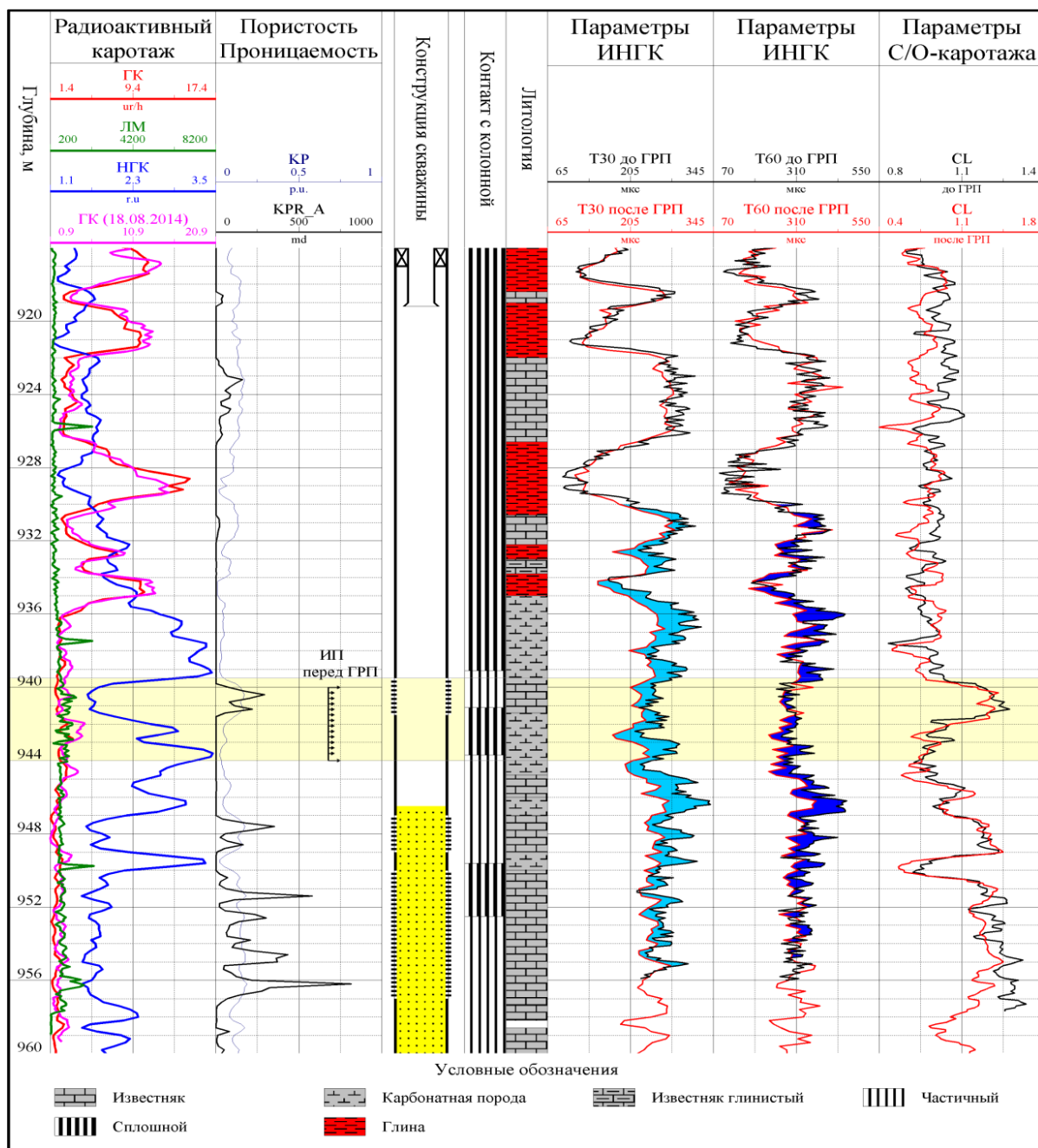
Рис. 5. Влияние маркированного проппанта на показания метода ИНГК
