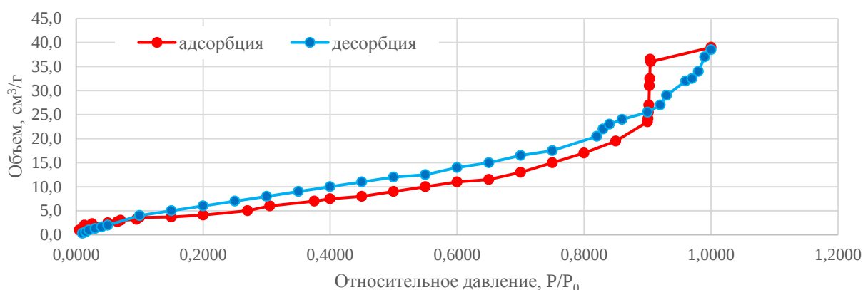
Рис. 4. Изотерма адсорбции–десорбции азота при 77 К (гидроуголь (акт. H 2 O 2 ))
