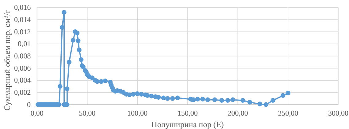
Рис. 3. Распределение пор по размерам: а) гидроуголь (250 °С, 2 ч); б) гидроуголь (акт. H 2 O 2 )
