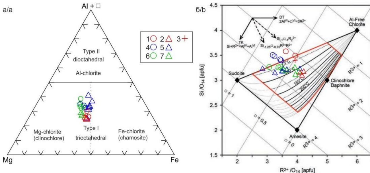
Рис. 3. Состав и оценка температуры кристаллизации хлоритов из пород экзоконтакта: а) классификация Mg-Al+Y-Fe (ф.е.) по [11]; б) диаграмма R^{2+} -Si (ф.е.) [12] с изотермами [13]. 1–3 – метааргиллиты: 1, 2 – обр. k 23 -78: 1 – матрикс, 2 – метакристаллы, 3 – обр. k 23 -82, матрикс; 4, 5 – силикатно-карбонатные метасоматиты, матрикс: 4 – обр. k 23 -80а, 5 – обр. k 23 -81; 6, 7 – скарнированный известняк, обр. k 23 -84: 6 – матрикс, 7 – стилолит
