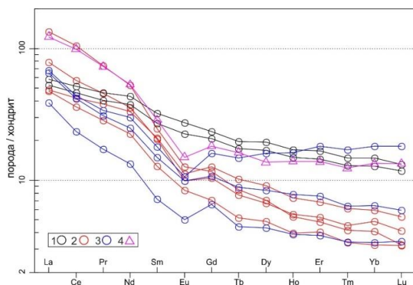
Рис. 6. Спектры распределения РЗЭ в габбро худолазовского комплекса и метаосадочных породах экзоконтакта, нормированные на хондрит [15]: 1 – габбро; 2 – метааргиллиты; 3 – силикатно-карбонатные метасоматиты; 4 – постархейский австралийский сланец (PAAS) [16]
