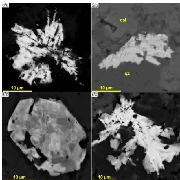
Рис. 4. BSE изображения главных акцессорных РЗЭ-содержащих минералов: а, б) розетковидные сростания кристаллов синхизита-(Ce) в силикатно-карбонатных метасоматитах: а) обр. k 23 -80а; б) обр. D 3 -16; в, г) РЗЭ-содержащий клинозоизит: в) идиоморфный неоднородный кристалл в силикатно-карбонатном метасоматите, обр. k 23 -81; г) сростание удлиненных кристаллов в метааргиллите, обр. 60-6
