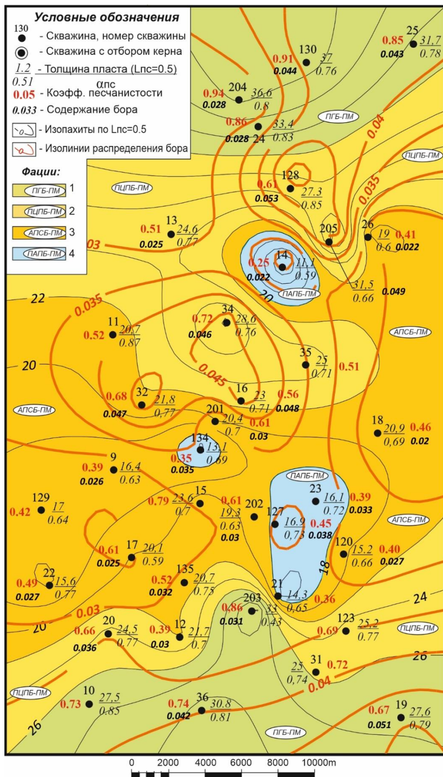
Рис. 3. Литолого-фациальная карта и характер распределения относительного содержания бора в пласте ХМ_2 одного из месторождений п-ва Ямал; фации: 1 – крупно-среднезернистых песков гребневых частей баров; 2 – среднезернистых песков центральных частей баров; 3 – средне-мелкозернистых песков и алевритов склоновых частей баров; 4 – песчано-алевритовых осадков подножий баров
