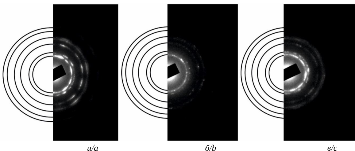
Рис. 4. Микродифракционные картины PdНЧ: а) PdНЧ–БГ; б) PdНЧ–Ц; в) PdНЧ–БГЦ Fig. 4. Microdiffraction patterns of PdNPs: а) PdNPs–BG; б) PdNPs–C; в) PdNPs–BGC
