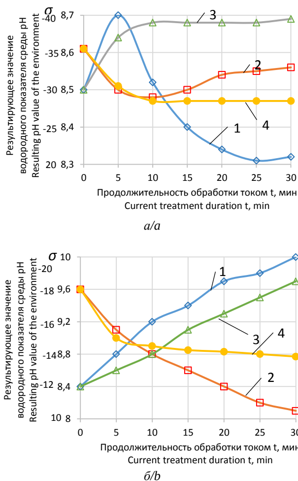
Рис. 1. Зависимость изменения величины pH и \sigma от продолжительности обработки током пластово-щелочной (а) и морской (б) вод. Величины pH и \sigma при напряжениях 100 В (1,2) и 20 В (3,4)
