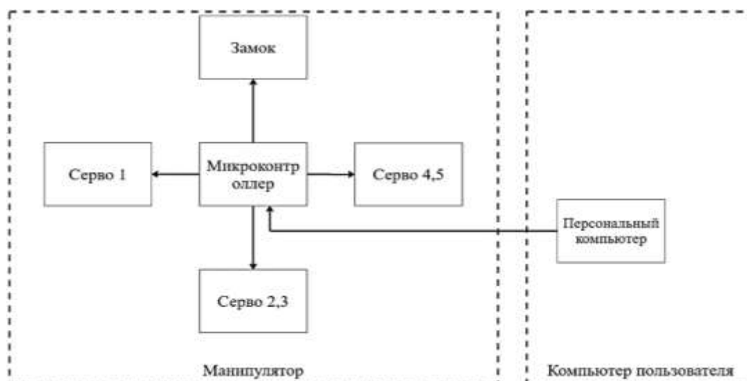
Рис. 1. Структурная схема
