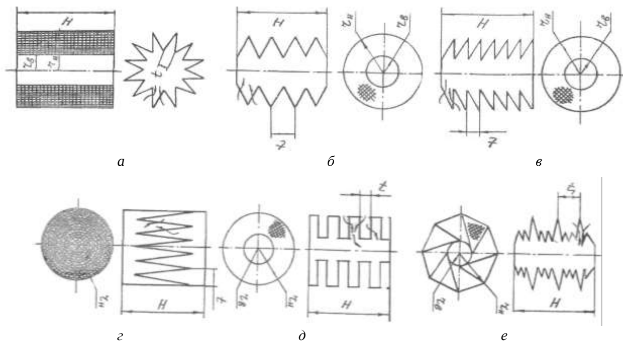
Рис. Типы фильтров с различными схемами укладки фильтрующих штор:
