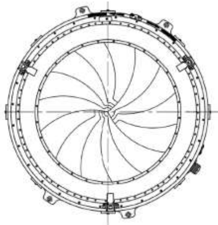
Рис. 3. Шторное устройство в закрытом состоянии
