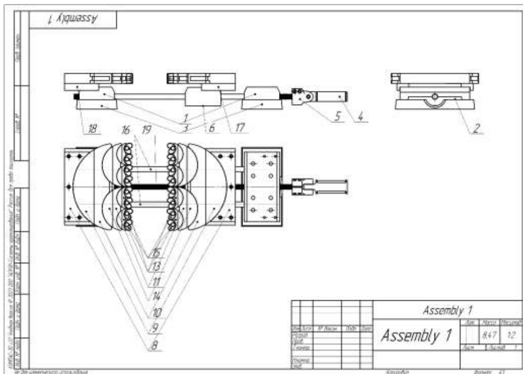
Рис. 1. Фрактальные тисы сборочный чертеж
