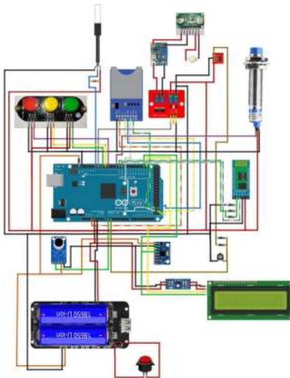
Рис. 2. Электрическая схема ГТН-01.01
