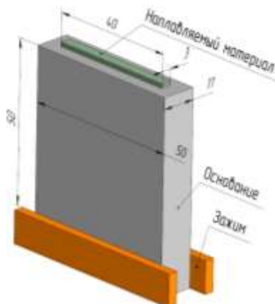
Рис. 1. Схема геометрии образца
