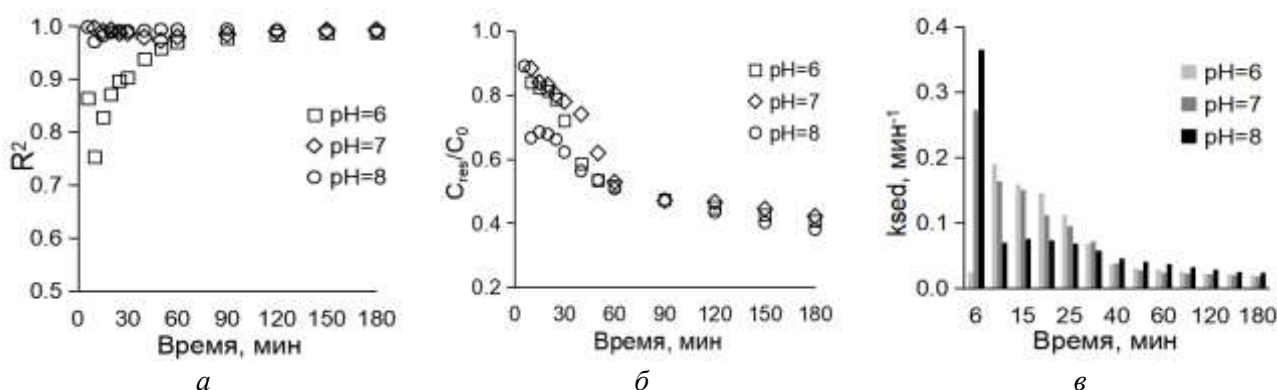
Рис. 1. Влияние времени седиментации на коэффициент детерминации R^2 (а), остаточную концентрацию частиц C_{\text{res}}/C_0 (б) и константу скорости осаждения k_{\text{sed}} (в) в воде при разном pH. Двухкратный эксперимент
