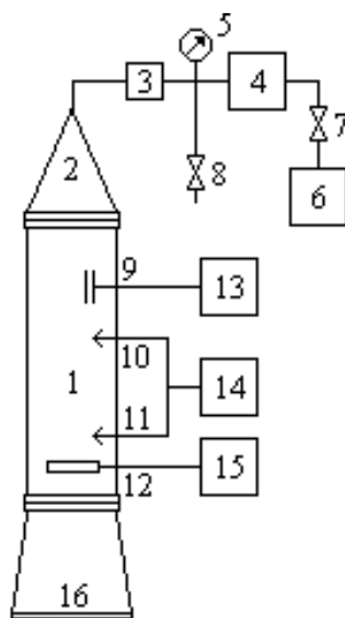
Рис. 1. Схема экспериментального прибора контроля и диагностики свойств композитных составов из низкосортных углей:
