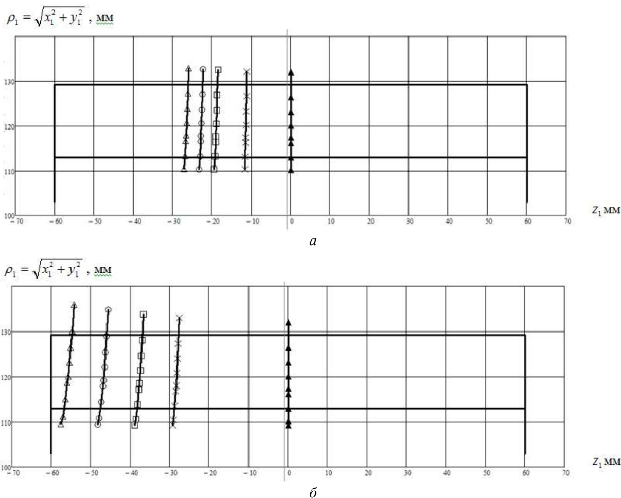
Рис. 3. Активные действующие линии в зацеплении при не параллельности: \eta = 0' ( \blacktriangle ); \eta = 3' ( \times ); \eta = 5' ( \square ); \eta = 6' ( \circ ); \eta = 7' ( \Delta )
