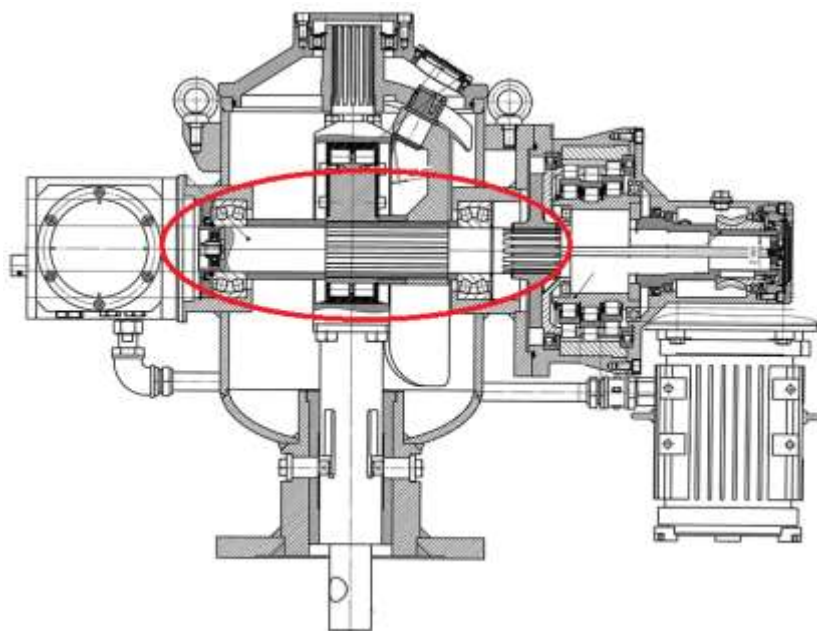
Рис. 1. Электропривод прямоходно-вращательный
