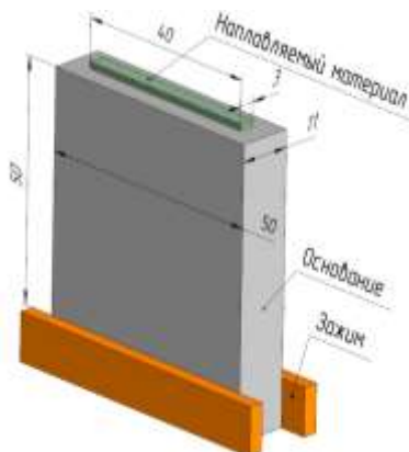
Рис. 1. Схема геометрии образца
