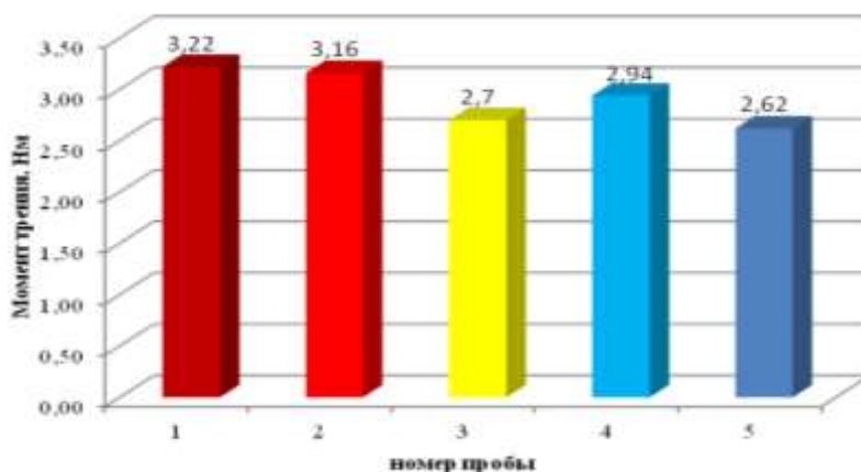
Рис. 1. Диаграмма соотношения моментов трения на устоявшемся режиме
