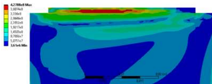
Рис. 3. Эквивалентные остаточные напряжения в результате наплавки
