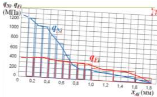
Рис. 1. Гистограммы удельных касательной q_F и нормальной q_N сил (МПа) на i -м участке пластины В. Абсцисса – расстояние от режущей кромки x_{Ai} (мм). Сталь 40Х–Т15К6, \gamma = +7^\circ ; v = 120 м/мин; a = s = 0,368 мм; b = 4 мм; c = 1,844 мм; c_1 = 0,922 мм; P_{y \text{ эксп}} = 1623 Н; P_{z \text{ эксп}} = 3061 Н; F_{\text{эксп}} = 2014 Н; N_{\text{эксп}} = 2837 Н
