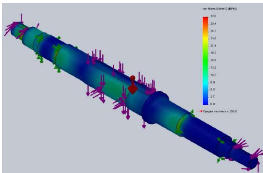
Рис. 2. Пример нагружения вала (в SolidWorks)
