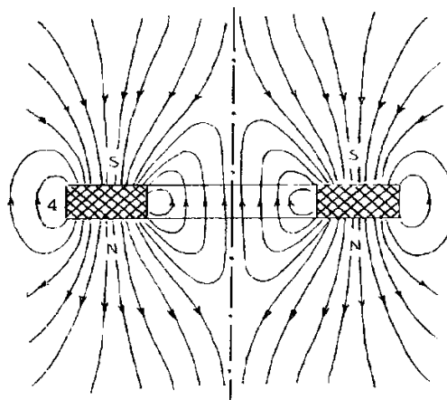
Рис. 5. Действие магнита
