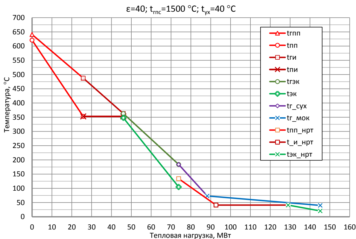
Рис. 3. Диаграмма изменения температур в поверхностях нагрева котла-утилизатора и теплутилизатора в зависимости от тепловой нагрузки
