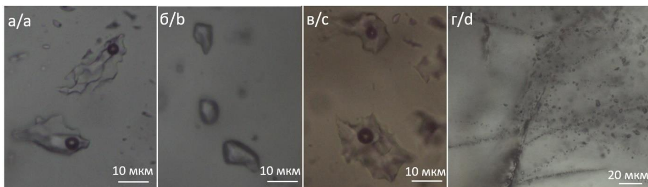
Рис. 4. Типы флюидных включений Аяхтинского месторождения: а) тип А, двухфазные ( \text{Ж}_{\text{H}_2\text{O}} + \text{Г}_{\text{CO}_2 \pm \text{CH}_4 \pm \text{N}_2} ); б) тип В, однофазные ( \text{Г}_{\text{CO}_2 \pm \text{CH}_4 \pm \text{N}_2} ); в) тип С, трехфазные ( \text{Ж}_{\text{H}_2\text{O}} + \text{Г} + \text{кр} ); г) система взаимно пересекающихся трещин, заполненных вторичными включениями
