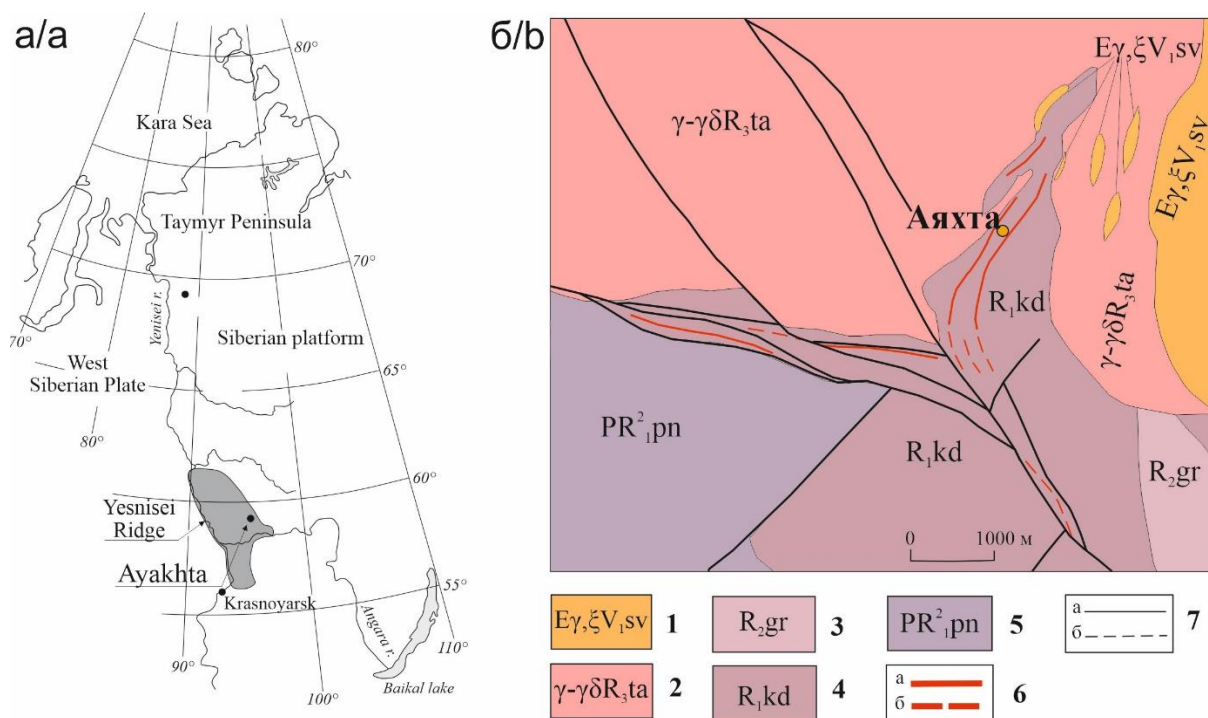
Рис. 1. а) географическое положение месторождения Аяхта; б) фрагмент геологической карты Аяхтинского рудного узла [33]. 1 – Средневогоровский комплекс щелочно-гранит-сиенитовый; 2 – Татарско-аяхтинский комплекс гранитовый; 3 – Горбилокская свита; 4 – Кординская свита; 5 – Пенченгинская свита; 6 – золоторудные минерализованные зоны (а – установленные, б – предполагаемые); 7 – разрывные нарушения (а – установленные, б – предполагаемые)
