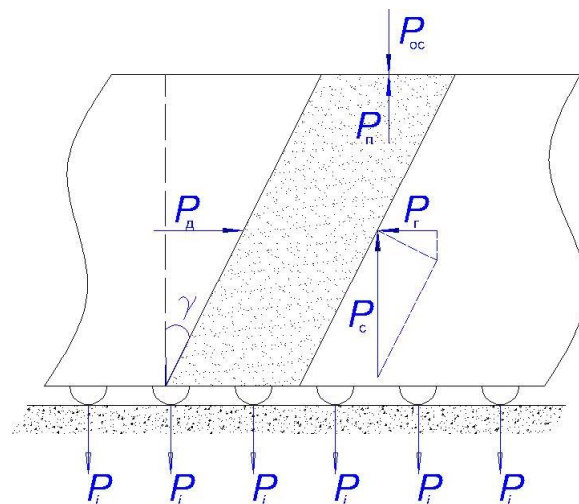
Рис. 6. Схема силового воздействия на наклонный алмазосодержащий штабик в процессе работы: P_d – дезориентирующее усилие, Н; P_c – реакция разрушаемой горной породы, Н; P_z – горизонтальная составляющая реакции разрушаемой горной породы, Н; \gamma – угол наклона штабика, град; P_{ос} – осевая нагрузка, даН; P_i – сила, действующая на резец, Н
