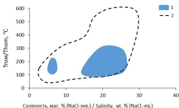
Рис. 6. Температура гомогенизации ( T_{\text{гом}} ) и соленость флюида месторождения Аяхта (1) и флюидов других месторождений золота Енисейского кряжа (2) – Олимпиада, Эльдorado, Советское, Герфед, Богунайское, Ведуга, Удереи, Панимба, Благодатное [12, 13, 19, 22, 27, 46–51]
