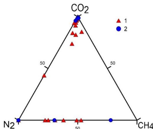
Рис. 5. Состав газовой фазы индивидуальных флюидных включений в кварце месторождения Аяхта (по результатам рамановской спектроскопии): 1 – тип А, двухфазные ( \text{Ж}_{\text{H}_2\text{O}} + \text{Г}_{\text{CO}_2 \pm \text{CH}_4 \pm \text{N}_2} ), 2 – тип В, однофазные ( \text{Г}_{\text{CO}_2 \pm \text{CH}_4 \pm \text{N}_2} ) включения
