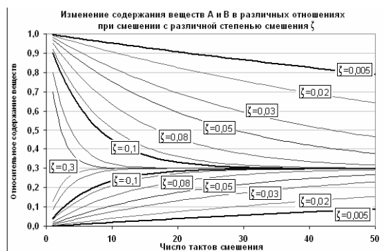
Рис. 9. График изменения содержания веществ при различной интенсивности смешения, отношение веществ 3/7
