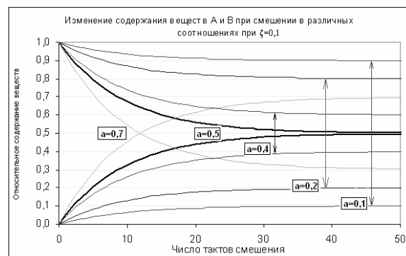
Рис. 8. График изменения содержания веществ при их различных соотношениях, степень смешения \zeta=0,1
