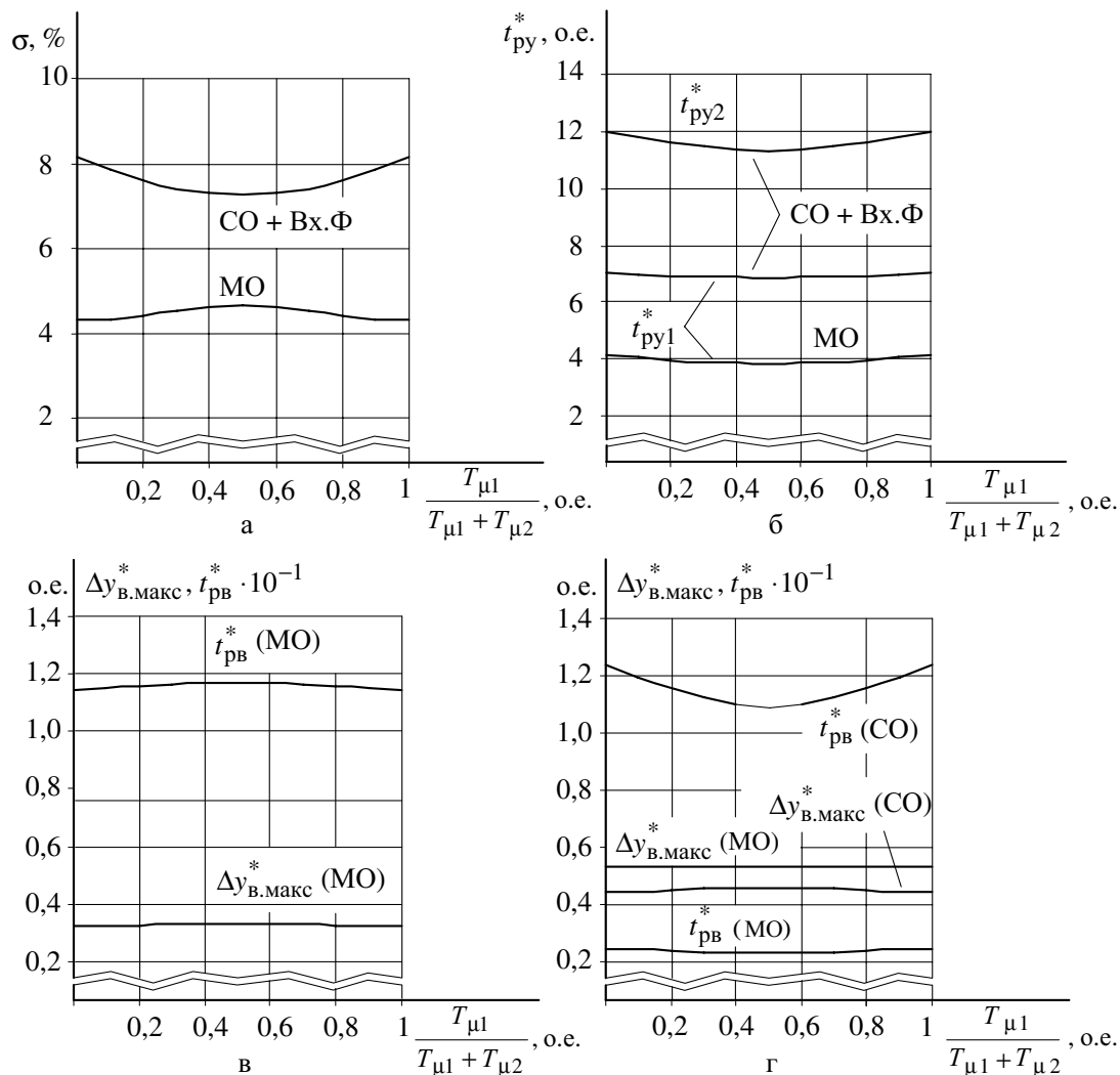
Рис. 1. Зависимости показателей качества обработки оптимизированным контуром ступенчатого управляющего и возмущающего z_3 воздействия от соотношения двух малых постоянных времени в прямом канале контура контура: а) б) и г) с интегрирующим звеном; в) с инерционными звеньями
