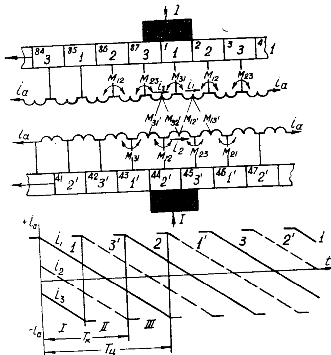
Рис. 1. Исходная схема и временная диаграмма коммутации ЭМУ.
