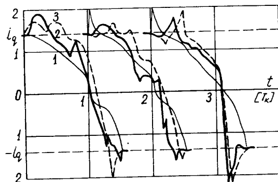
Рис. 2. Кривые тока коммутируемых секций поперечной цепи ЭМУ. 1 — расчет, 2,3 — опыт для переменного и постоянного тока.
