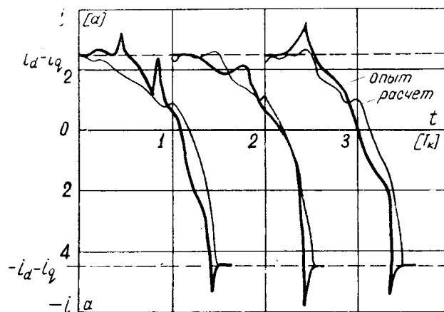
Рис. 3. Кривые тока коммутируемых секций продольной цепи ЭМУ.
