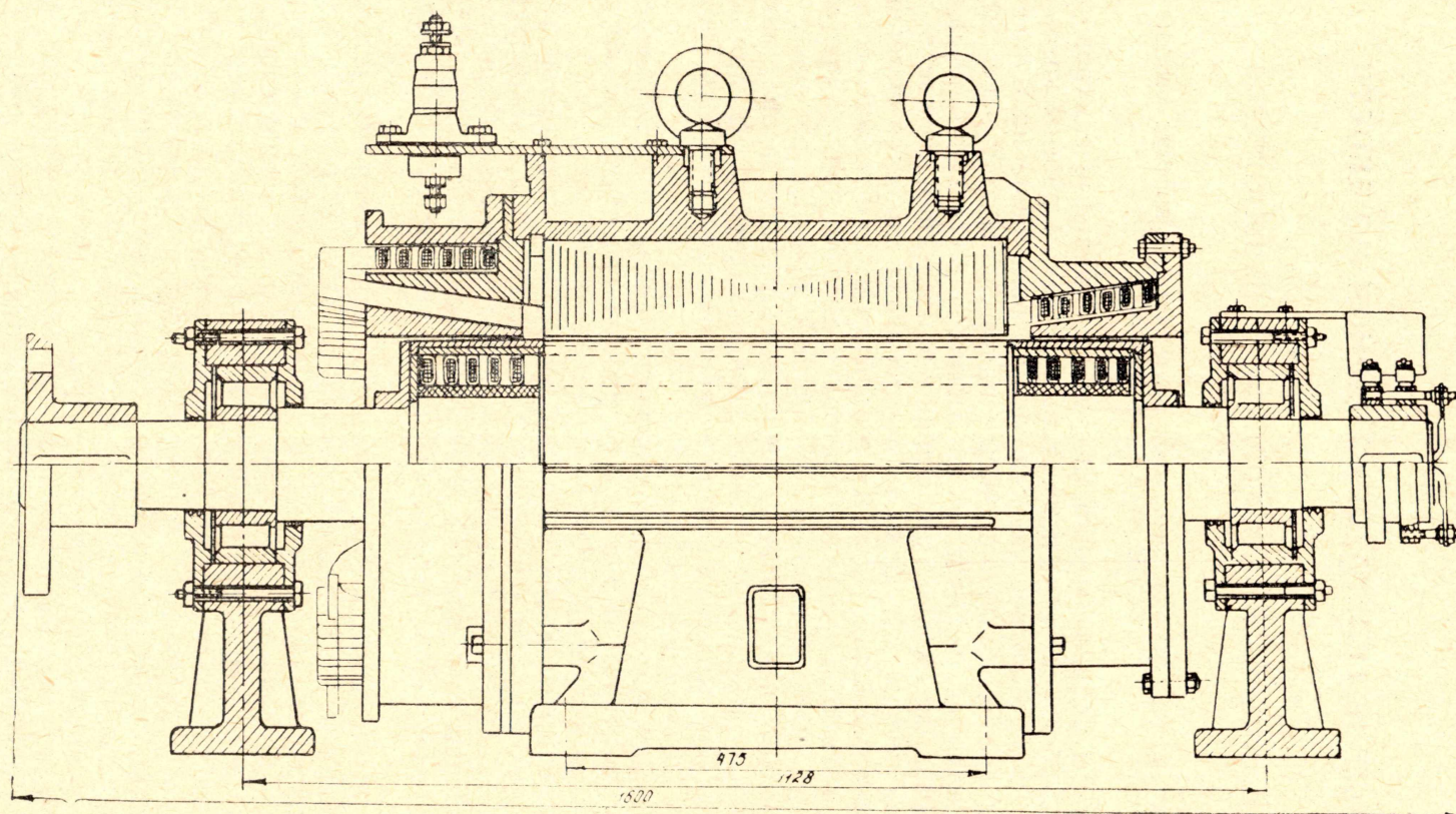
Р и с. 1. Общий вид ударного генератора в разрезе.
