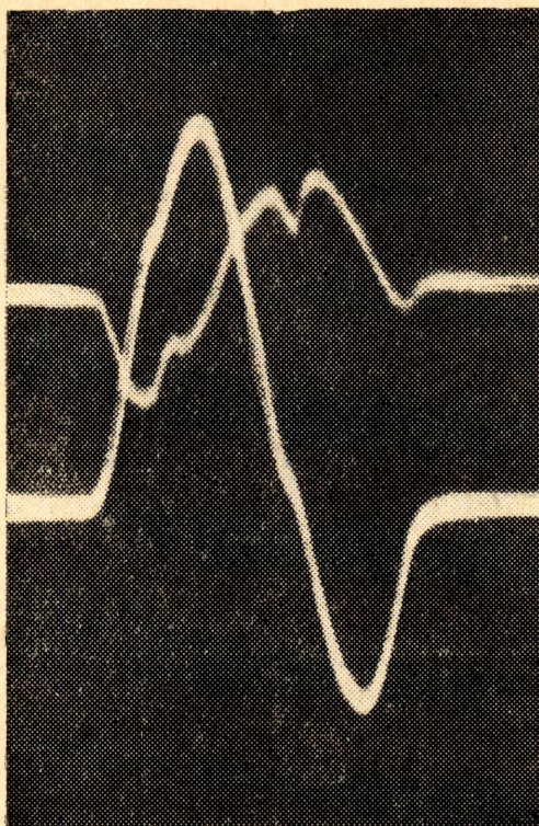
Р и с. 5. Осциллограммы тока возбуждения и ударного тока генератора.
