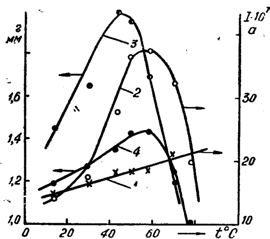
Рис. 2. Зависимость глубины анодного зубца свинца в 0,1 M растворе NH 4 Cl (кривые 1, 2) предельного радиуса (кривая 3) и среднего во времени радиуса капли амальгамы аммония (кривая 4) от температуры. Кривая 1— 2 \cdot 10^{-5} г-ион/л Рb 2+ , без ЭАА; кривая 2— 2 \cdot 10^{-6} г-ион/л Рb 2+ , при наличии ЭАА. Условия опыта V=10 мл; τ=5 мин; рН=8.
