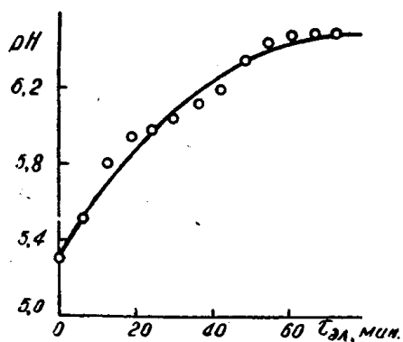
Рис. 1. Изменение рН раствора 1 M NH 4 Cl в течение электролиза при наличии ЭАА. Объем раствора V=15 мл; t=18°C.
