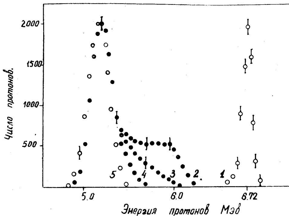
Рис. 7. Энергетическое распределение протонов с энергией 6,72 МэВ после прохождения монокристалла NaCl под различными углами относительно направления [100] 0^\circ — 2, 0,6^\circ — 3, 1,2^\circ — 4, 6^\circ — 5
