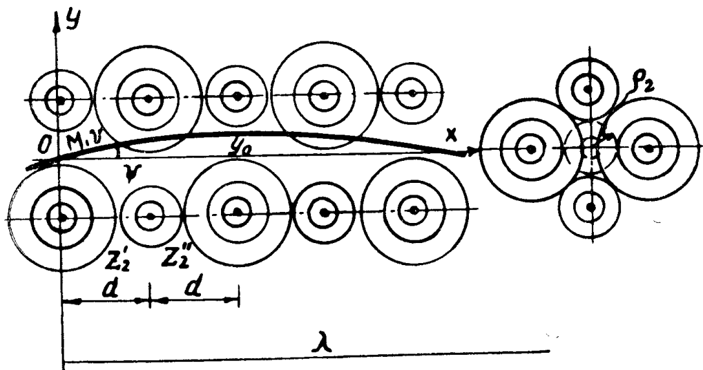
Рис. 1. Структура канала [100] в простой кубической решетке.
