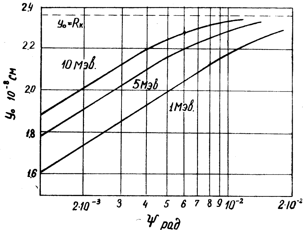
Рис. 4. Амплитуда колебаний траектории протона в канале [100] КВг в зависимости от угла влета протона в канал при различных значениях энергии протонов
