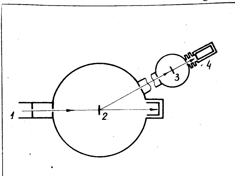
Рис. 6. Схема экспериментальной установки
