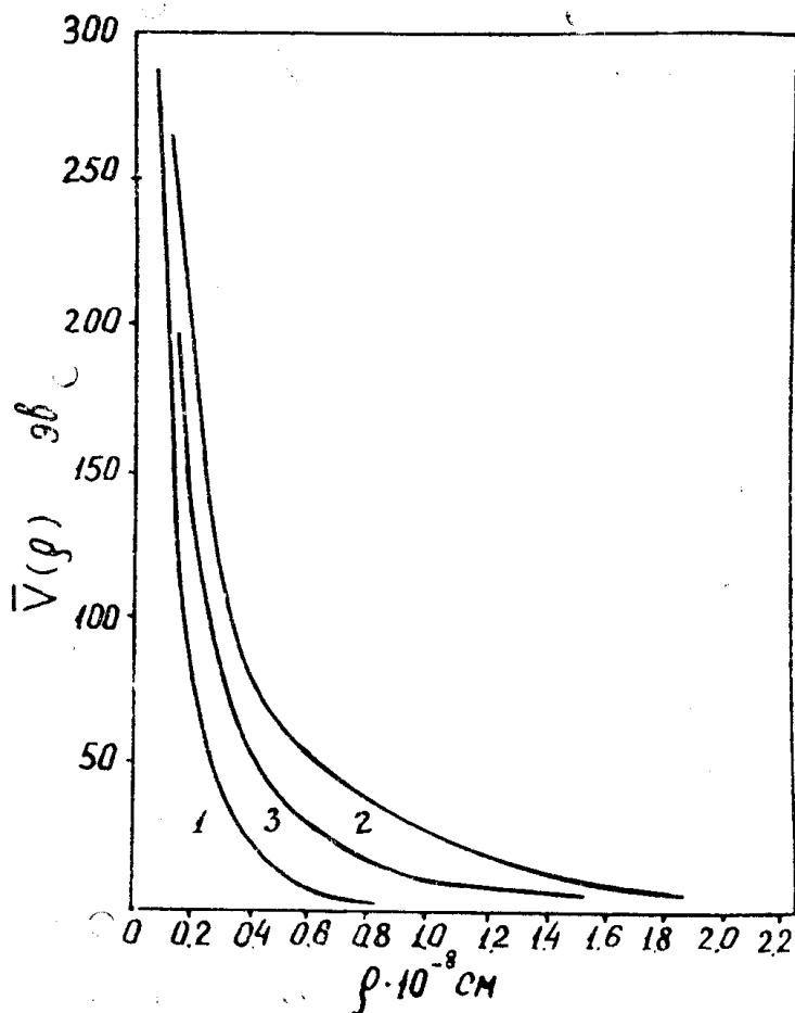
Рис. 2. Средние потенциалы V(\rho) для рядов [100] в KBr. Здесь и на следующем рисунке приняты следующие обозначения:
