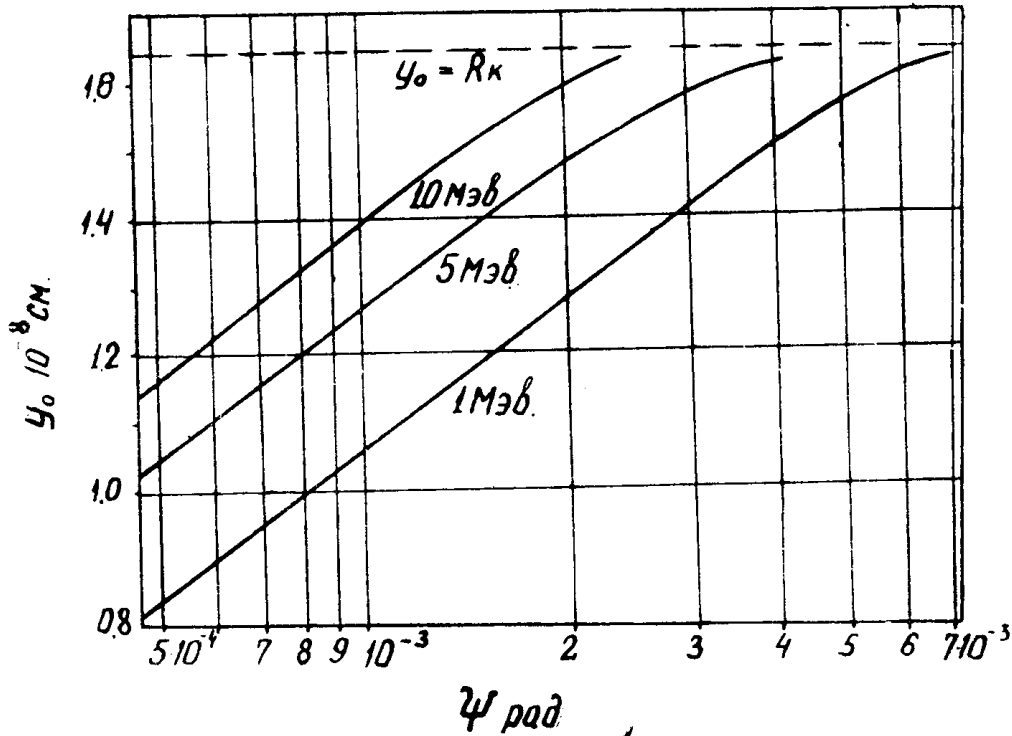
Рис. 5. Амплитуда колебаний траектории протона между плоскостями (100) КВг в зависимости от угла влета при различных значениях энергии протонов
