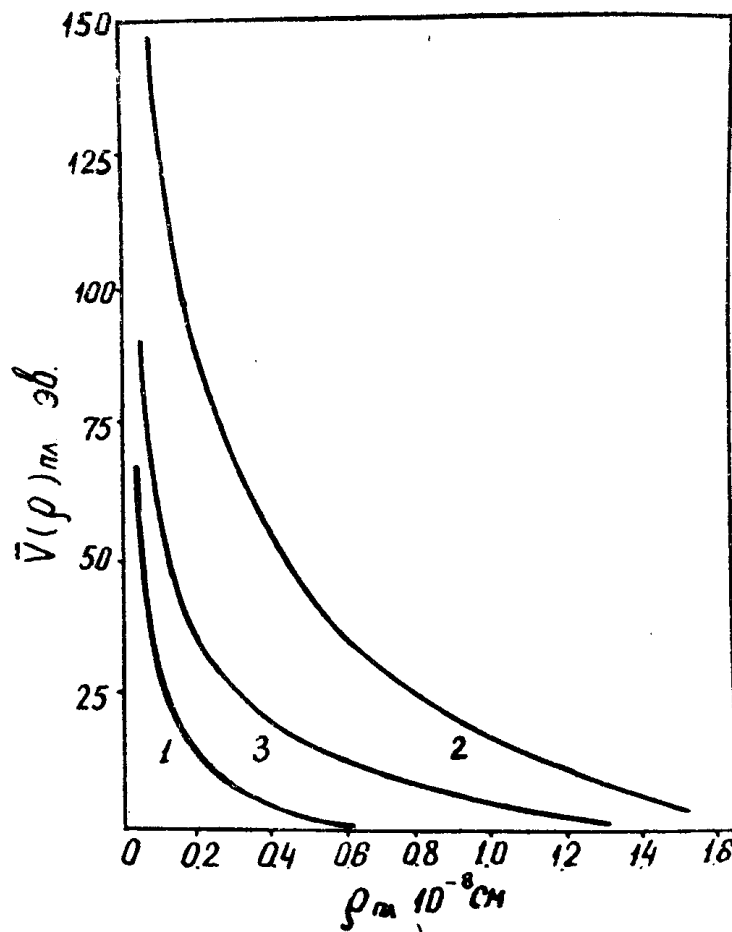
Рис. 3. Средние потенциалы \bar{V}(\rho)_{пл} для плоскостей (100) в КВг
