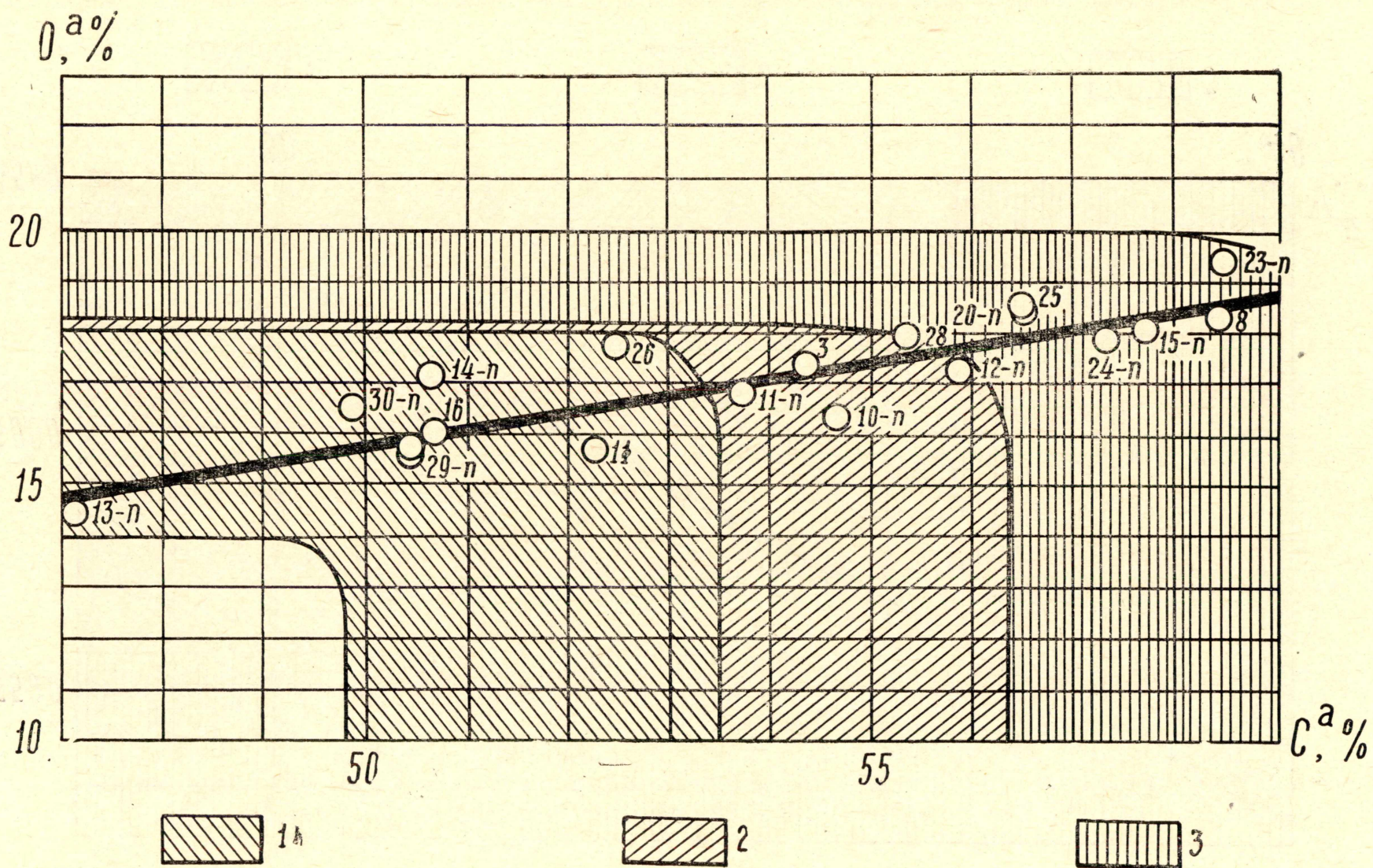
Рис. 2. Элементарный состав углей в зависимости от их петрографического состава. Условные обозначения те же
