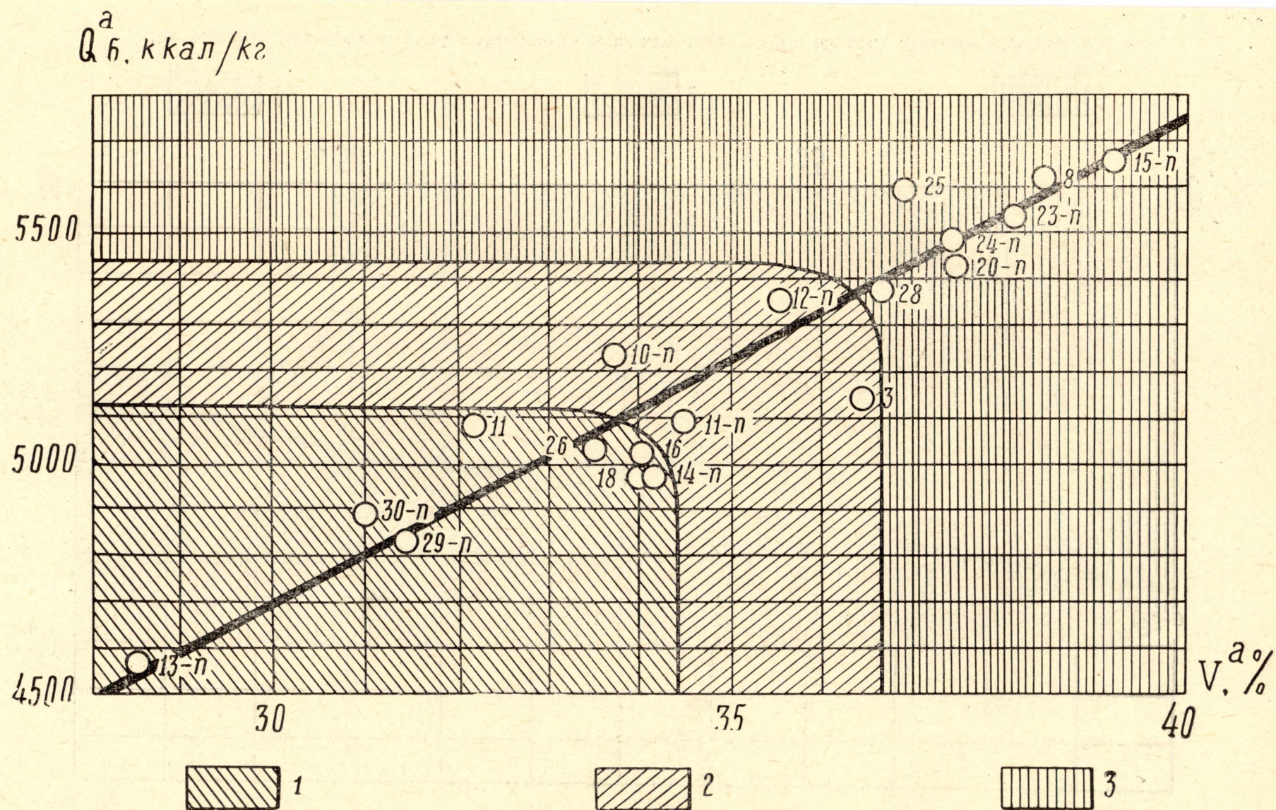
Рис. 1. Зависимость теплотворной способности и выхода летучих от петрографического состава углей. Условные обозначения: 1 — клареновый тип углей; 2 — клареново-дюреновый и дюрено-клареновый типы углей; 3 — сапропелито-гумитовый тип углей
