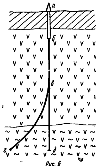
Рис. 6. Схема бурения двухствольной скважины
