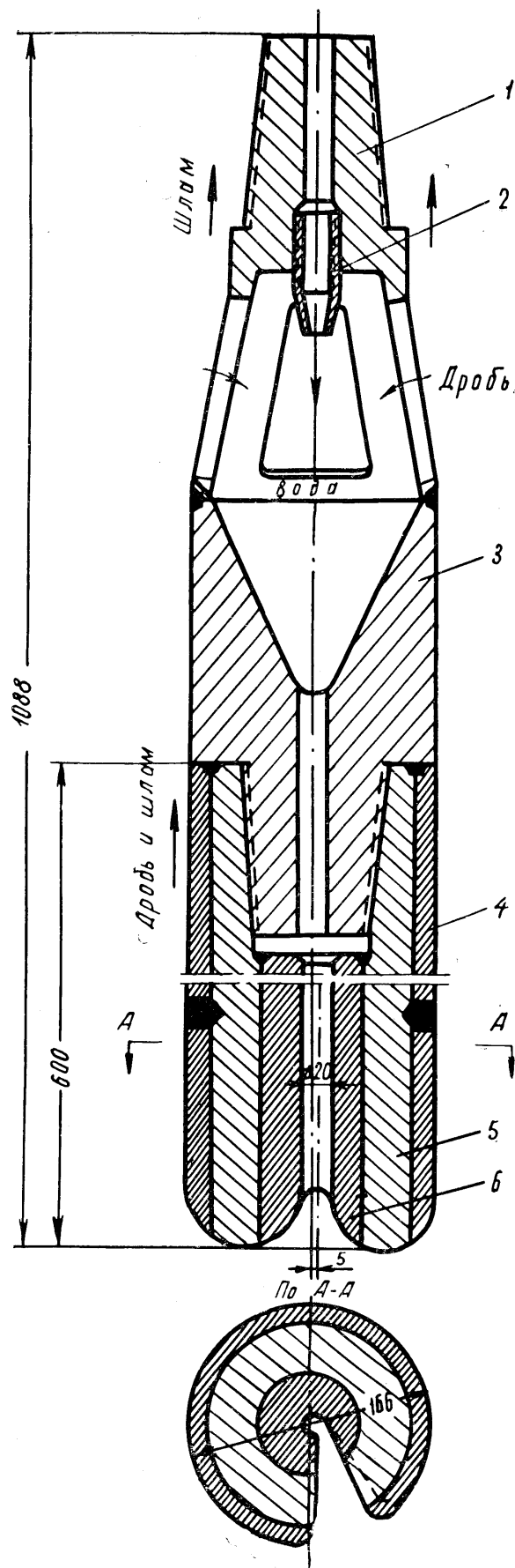
Рис. 4. Дробовая коронка для бурения сплошным забоем: 1 — верхняя часть корпуса; 2 — гидравлическая насадка; 3 — нижняя часть корпуса; 4 — коронка; 5 и 6 — втулки
