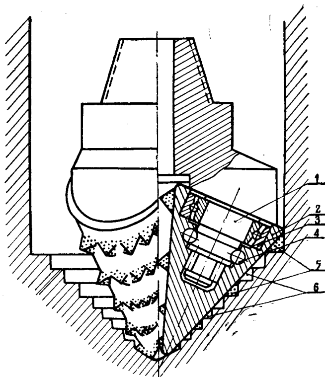
Рис. 5. Шарошечное ступенчатое долото: 1 — цапфа; 2 — шарошка; 3 — радиально-упорный подшипник; 4 — шариковый замковый подшипник; 5 — зубья шарошек; 6 — ступени забоя
