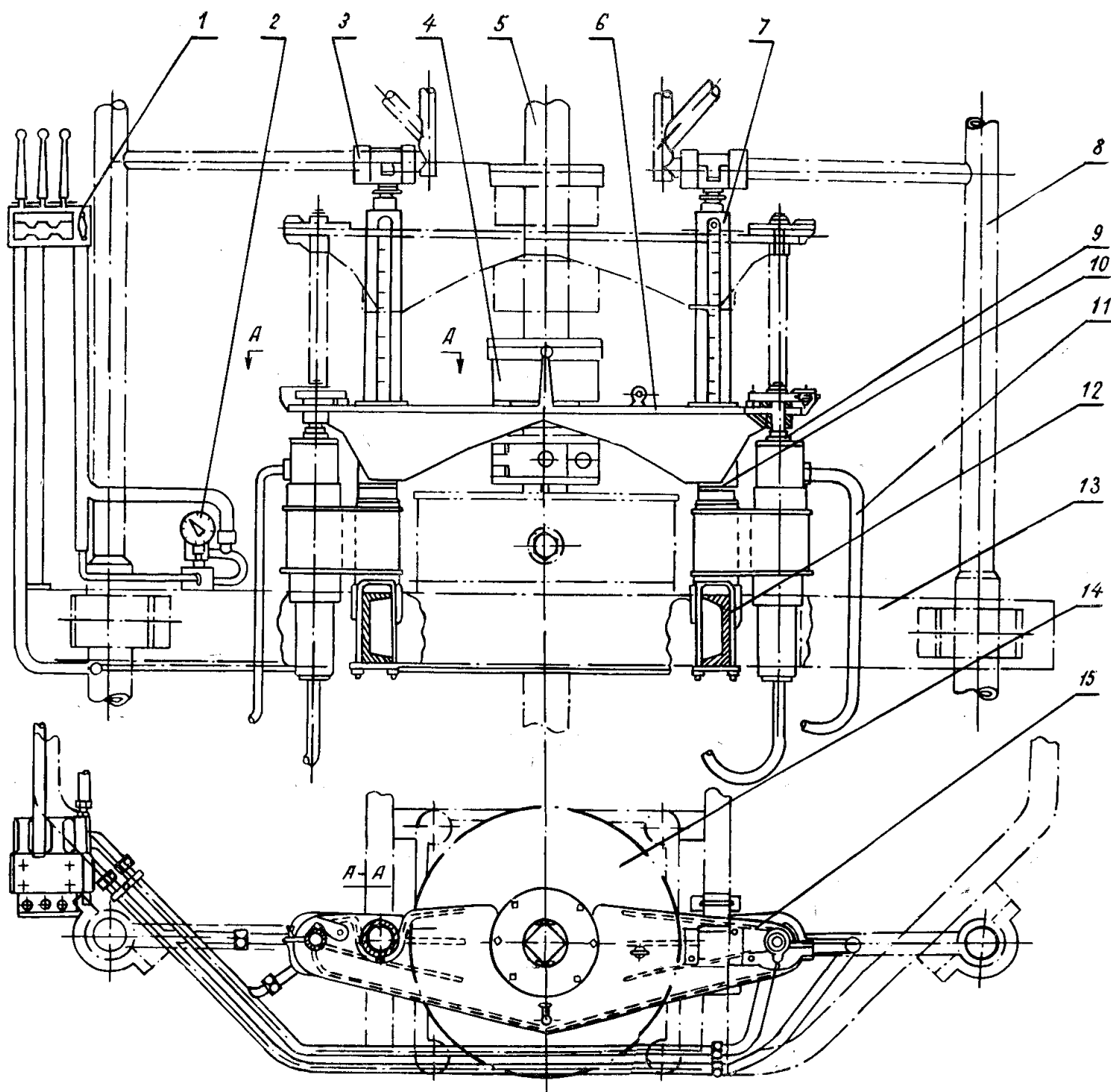
Рис. 3. Схема гидроснабжения к установке УРБ-3АМ:
