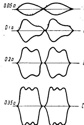
Рис. 2. Зависимость огибающей второй гармоники от величины тока подмагничивания
