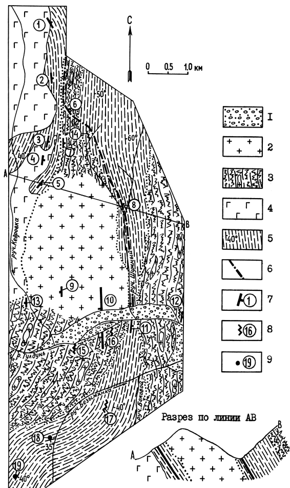
Рис. 1. Схема геологического строения Кедровского рудного поля (составлена с использованием материалов В.А. Загоскина и Э.М. Мулюкова): 1) речные пойменные и террасовые отложения; 2, 3) очагово-купольная структура палеозоя: 2) гранодиорит, кварцевый диорит, 3) альмандин-биотитовые плагиогнейсы, плагиомигматиты с мелкими телами кварцевого диорита; 4) габбро, габбро-диорит Кедровского массива; 5) графит-содержащие биотит-полевошпат-кварцевые, двуслюдяные полевошпат-кварцевые песчано-алевросланцы с горизонтами известняков кедровской свиты; 6) Главное нарушение; 7) участки локализации золоторудных кварцевых жил: Жиганских (1), Пинегинских (2), Осинových (3), Промежуточных (4), Шаманских (5), Штурмовых (6), Параллельной (7), Шумной (8), Баргузинской-II (9), Баргузинской-I (10), Майской (11), Безымянной (12), Кедровской (13); 8) участки локализации аполанцевых и апомигматитовых метасоматических залежей березитоидов: верховьев руч. Шумный (14), устья руч. Кедровки (15), устья руч. Шумный (16), Нижней Безымянки (17); 9) участки локализации кварцевого жильно-прожилкового оруденения в зонах рассланцевания: первый (18), второй (19)
