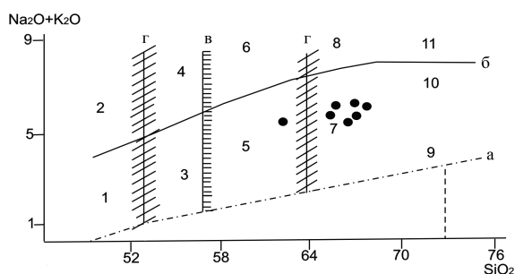
Рис. 2. Положение магматических пород зрелой очагово-купольной структуры Кедровского золоторудного месторождения в координатах SiO 2 – (Na 2 O+K 2 O): а) нижняя граница распространения химических составов магматических горных пород, б) нижняя граница распространения химических составов умеренно щелочных магматических горных пород, в) граница распространения кварца >5 %, г) границы разделения магматических горных пород на группы с «полями неопределенности». Области распространения: 1) габброидов, 2) умеренно щелочных габброидов, 3) диоритов, 4) умеренно щелочных диоритов-монцонитов, 5) кварцевых диоритов, 6) умеренно щелочных кварцевых диоритов – кварцевых монцонитов, 7) гранодиоритов, 8) кварцевых сиенитов, 9) низкощелочных гранитов, 10) гранитов, 11) умеренно щелочных гранитов. Границы распространения областей пород заимствованы из [23]
