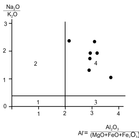
Рис. 3. Положение магматических пород зрелой очагово-купольной структуры Кедровского золоторудного месторождения в координатах Na 2 O/K 2 O – Al 2 O 3 /(MgO+FeO+Fe 2 O 3 ). Серия, глинозёмистость: 1) калиевая, высокоглинозёмистые, 2) калиево-натриевая, высокоглинозёмистые, 3) калиевая, весьма высокоглинозёмистые, 4) калиево-натриевая, весьма высокоглинозёмистые. Границы полей серий и коэффициента глинозёмистости заимствованы из [23]
