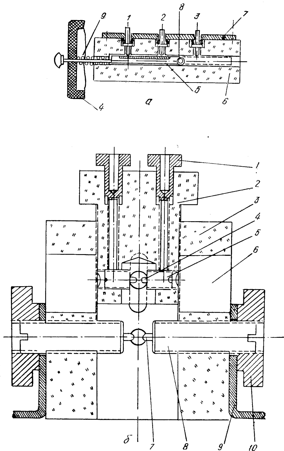
Рис. 2. Конструкция коммутаторов 1 а — ударный переключатель — разрядник, б — четырехэлектродный искровой разрядник.
