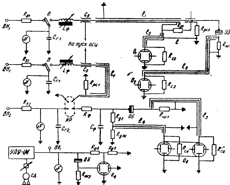
Рис. 1. Схема установки для исследования возбуждения химических процессов электрическим полем
