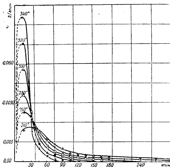
Рис. 6. Изменение скорости реакции \text{TiBr} + \text{HCl} = \text{TiCl} + \text{HBr} во времени.
