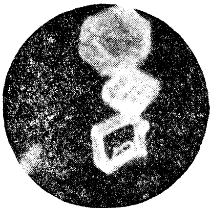
Рис. 9. Кристаллы бромида таллия до реакции X120.
