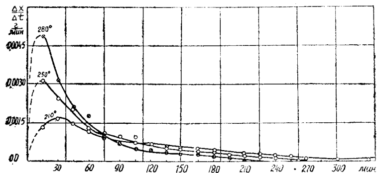
Рис. 4. Изменение скорости реакции \text{AgBr} + \text{HCl} = \text{AgCl} + \text{HBr} во времени.
