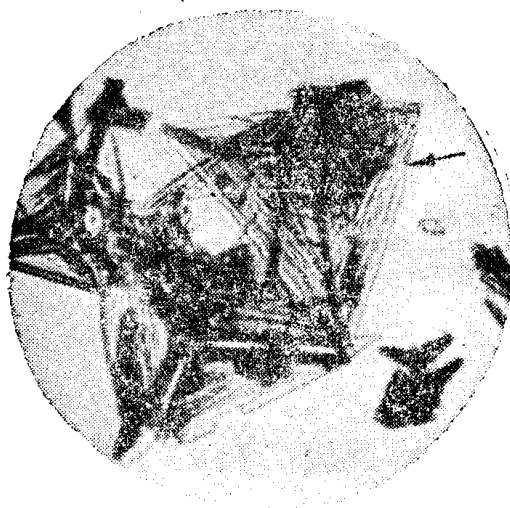
Рис. 13. Тетраэдрические кристаллы бромида меди с vicinalными гранями. Стрелкой указан обрыв спиралей роста X300.
