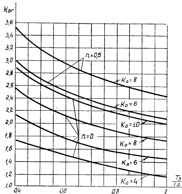
Рис. 2. Оптимальные коэффициенты форсированного развозбуждения
