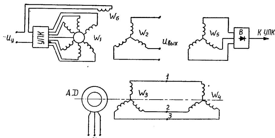
Рис. 1. Принципиальная схема ЭМУ-РЧ
