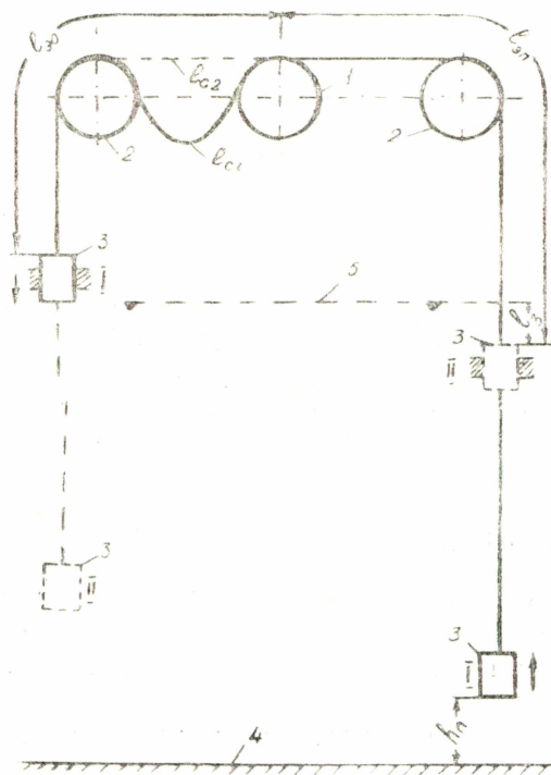
Рис. 1. Принципиальная механическая схема подъемной установки: 1 — органы навивки; 2 — направляющие шкивы; l_{с0}, l_{сн} — длина каната, воспринимающая экстренную нагрузку со стороны опускающегося и поднимающегося сосудов.
