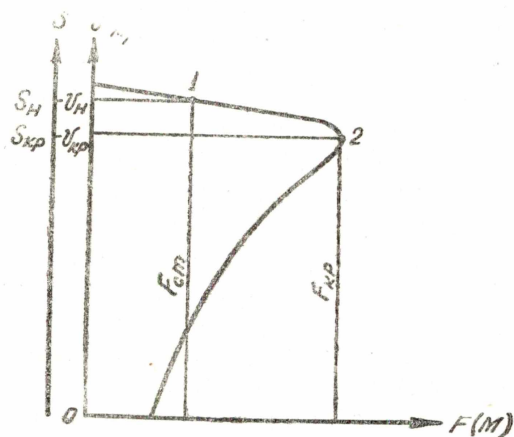
Рис. 2. Естественная механическая характеристика асинхронного подъемного двигателя.
