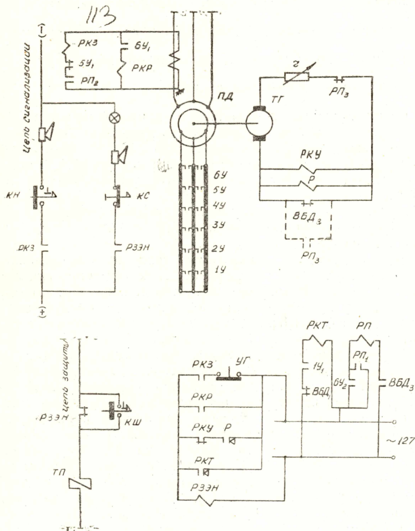
Рис. 4. Принципиальная схема защиты от обрыва подъемного каната экстренными нагрузками: ПД—подъемный двигатель; ТГ—тахогенератор; ВБД 1 , ВБД 2 , ВБД 3 —контакты индуктивного выключателя; ТП—контактор предохранительного тормоза; КС—кнопка сброса сигнала.
