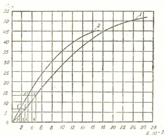
Рис. 3. Диаграмма испытания каната на разрыв: 1—канат новый (до навески); 2—канат, снятый с эксплуатации по признаку обрыва 5% проволок на шаге свивки (проработал 16,5 мес.).
