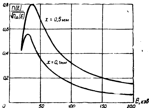
Рис. 3. Изменение отношения сигнал/шум из-за того, что в мишени поглощается только часть падающего на торцевое стекло излучения.
