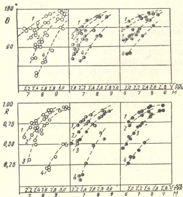
Рис. 1. Зависимость модуля коэффициента отражения R и фазового угла \Theta от числа маха M , частоты зондирующего излучения f для начальных давлений аргона p_0=2,5 и 10 мм рт.ст. 1— f=200 мГц, 2— f=452 мГц, 3— f=1000 мГц, 4— f=2000 мГц \circ , \bullet , \bullet — p_0=2,5 и 10 мм рт.ст.
