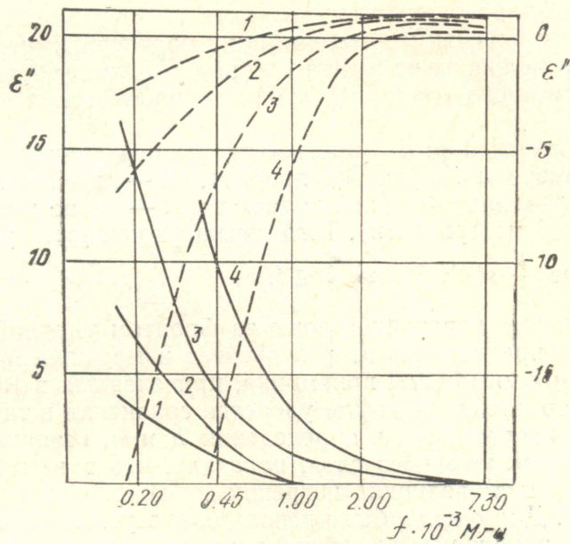
Рис. 2. Зависимость действительной \epsilon' и мнимой \epsilon'' частей комплексной диэлектрической проницаемости от частоты f при p_0 = 2 мм рт. ст. в аргоне. 1 — V = 2,2 км/сек, — — — \epsilon'' \epsilon' 2 — V = 2,4 км/сек, 3 — V = 2,6 км/сек, 4 — V = 2,8 км/сек
