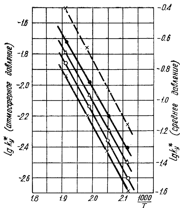
Рис. 1. Температурная зависимость эффективной константы скорости процесса: ———— давление — атмосферное, ———— фиктивная линейная скорость x — 0,295 см/сек, o — 0,590 см/сек, \Delta — 0,885 см/сек, \bullet — 1,475 см/сек, ———— давление — среднее
