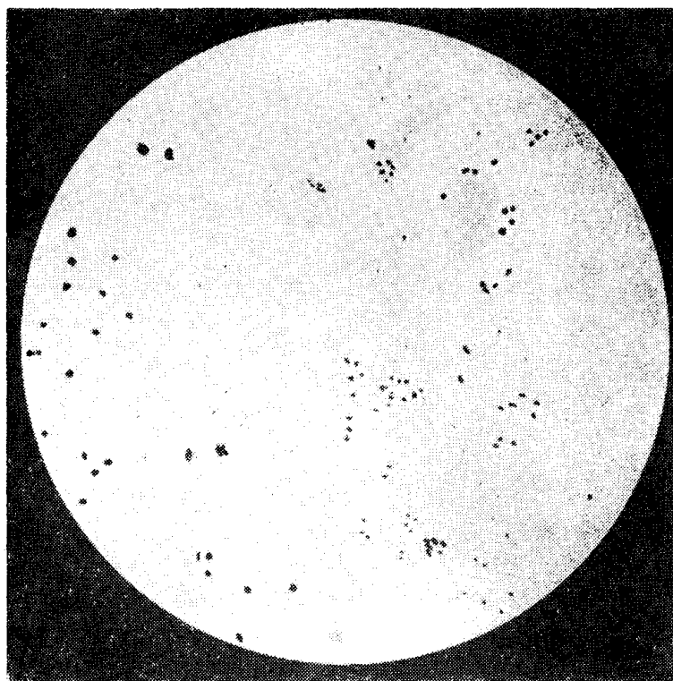
Рис. 3. Неметаллические включения стали ШХ-15, выплавленной при давлении 10 ат. ст.
