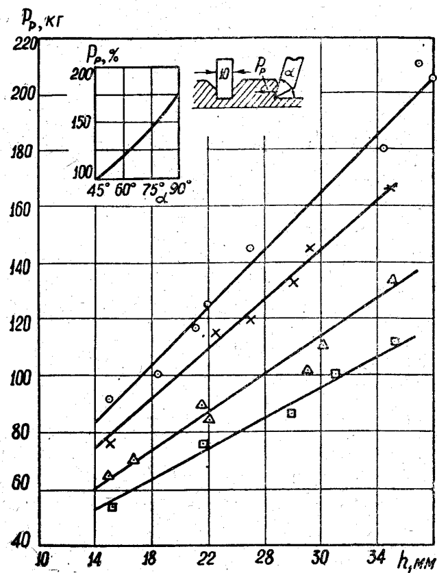
Рис. 2. Зависимость силы P_p резания мерзлого суглинка на глубине 1 м ( t = -3,3^\circ\text{C} ) от толщины стружки h и угла резания \alpha : 1— 45^\circ ; 2— 60^\circ ; 3— 75^\circ ; 4— 90^\circ
