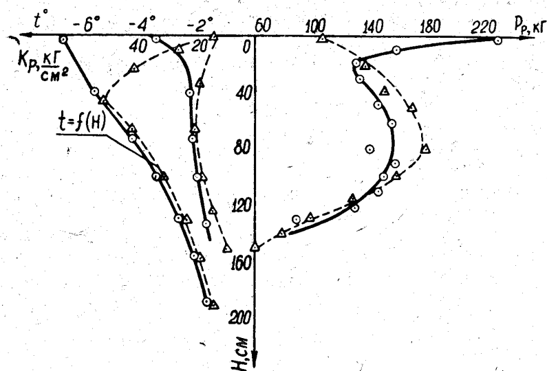
Рис. 1. Изменение температуры t , силы резания P удельной силы резания K_p по слою промерзания суглинка H при резании одиночным резцом с \alpha = 75^\circ , b = 10 мм, h = 25 мм: — 2/IV 1968 г. (число ударов ударника ДорНИИ C=58 , температура воздуха -15^\circ\text{C} ); --- 4/IV 1968 г. ( C = 25 , t_{\text{возд}} = -1,5^\circ\text{C} )
