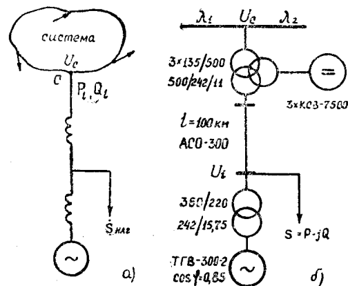
Рис. 1. Схема промежуточной системы
