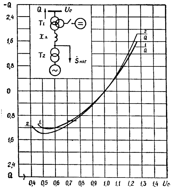
Рис. 2 а. Обобщенные статические характеристики промежуточной системы
