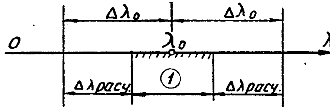
Рис. 2. \lambda_0 + \Delta\lambda_0 — номинальное значение перемещения конца пружины и допуск, установленные проектировщиком; 1 — область возможных отклонений истинного номинального значения перемещения конца пружины от значения \lambda_0 , установленного проектировщиком; \pm\lambda_{0расч} — допуск, исходя из которого следует определять допуски на значения параметров
