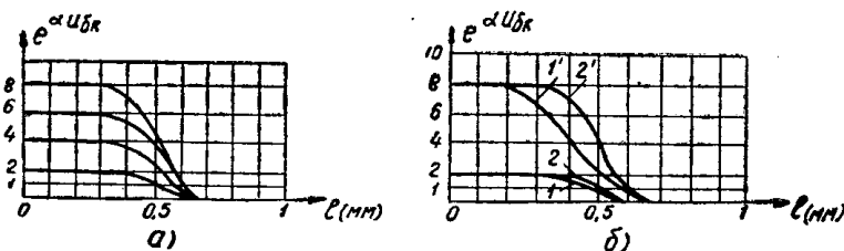
Рис. 1.— На рис. 1, а — кривые распределения e^{aU_{бк}} по l при U_t = 0,5 в, a = 50 мк, \rho = 10^5 ом·см в зависимости от M , где M = 2 + \beta Q / j_s . Линия переключения ячеек сканистора проходит при e^{aU_{бк}} = 1 . (точка переключения ячейки сканистора запаздывает тем больше, чем выше освещенность ее). На рис. 1, б — зависимость l^{aU_{бк}} при a = 20 мк, \rho = 10^5 ом·см. Кривые 1 и 2 при M = 2 и кривые 1' и 2' при M = 8 с учетом и без учета поперечного сопротивления базовой области. (Увеличение поперечного сопротивления базовой области влечет за собой расширение зоны переключения ячейки)
