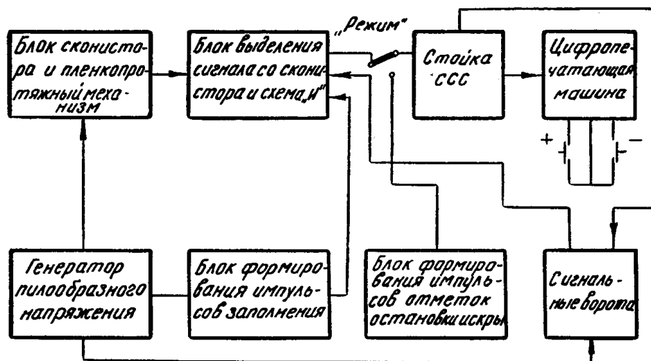
Рис. 2. Блок-схема установки
