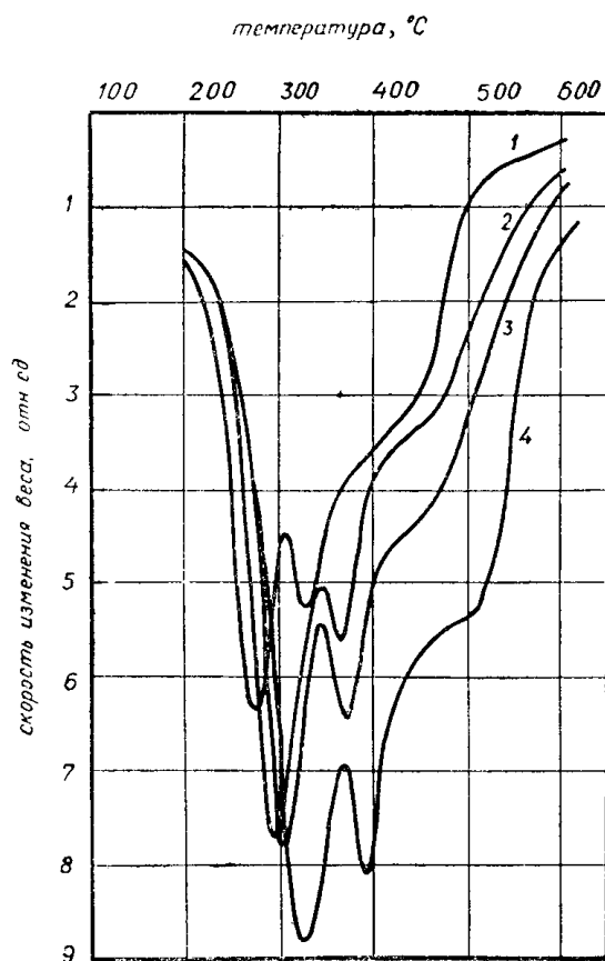
Рис. 1. Влияние окиси железа на скорость изменения веса при термическом разложении торфа. 1 — исходный торф, 2 — торф + 20% окиси железа, 3 — торф + 30% окиси железа, 4 — торф + 50% окиси железа.
