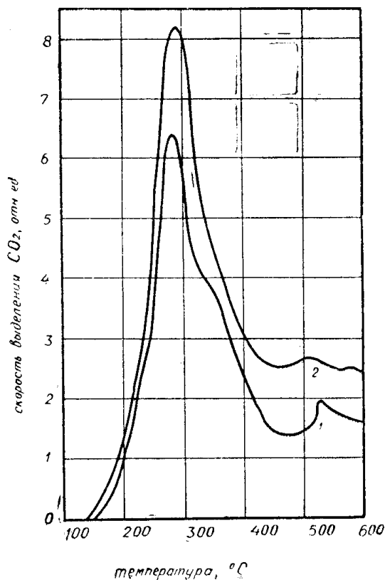
Рис. 3. Влияние окиси железа на скорость выделения \text{CO}_2 при термическом разложении торфа. 1 — исходный торф, 2 — торф + 30% окиси железа
