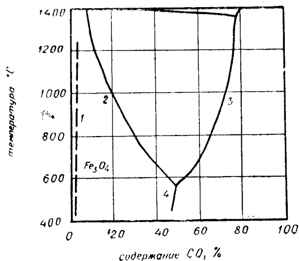
Рис. 2. Диаграмма равновесий окислов железа газовой фазой из \text{CO} и \text{CO}_2
