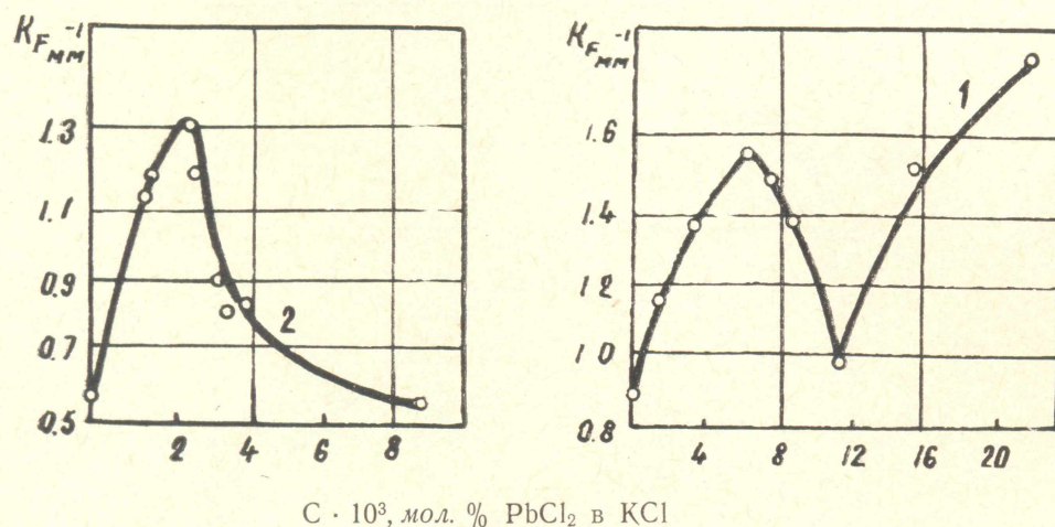
Рис. 4. Зависимость коэффициента поглощения в максимуме ( \lambda = 560 мкм) F -полосы от концентрации примеси PbCl_2 в KCl при комнатной температуре; 1 — для «растворных», 2 — для «расплавных» монокристаллов
