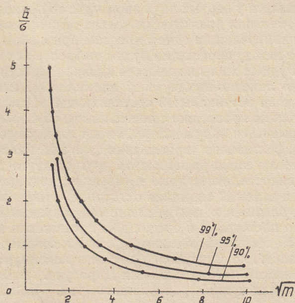
Рис. 1. Характеристика обнаружения аномалий по критерию Котельникова (А. А. Никитин и др.)
