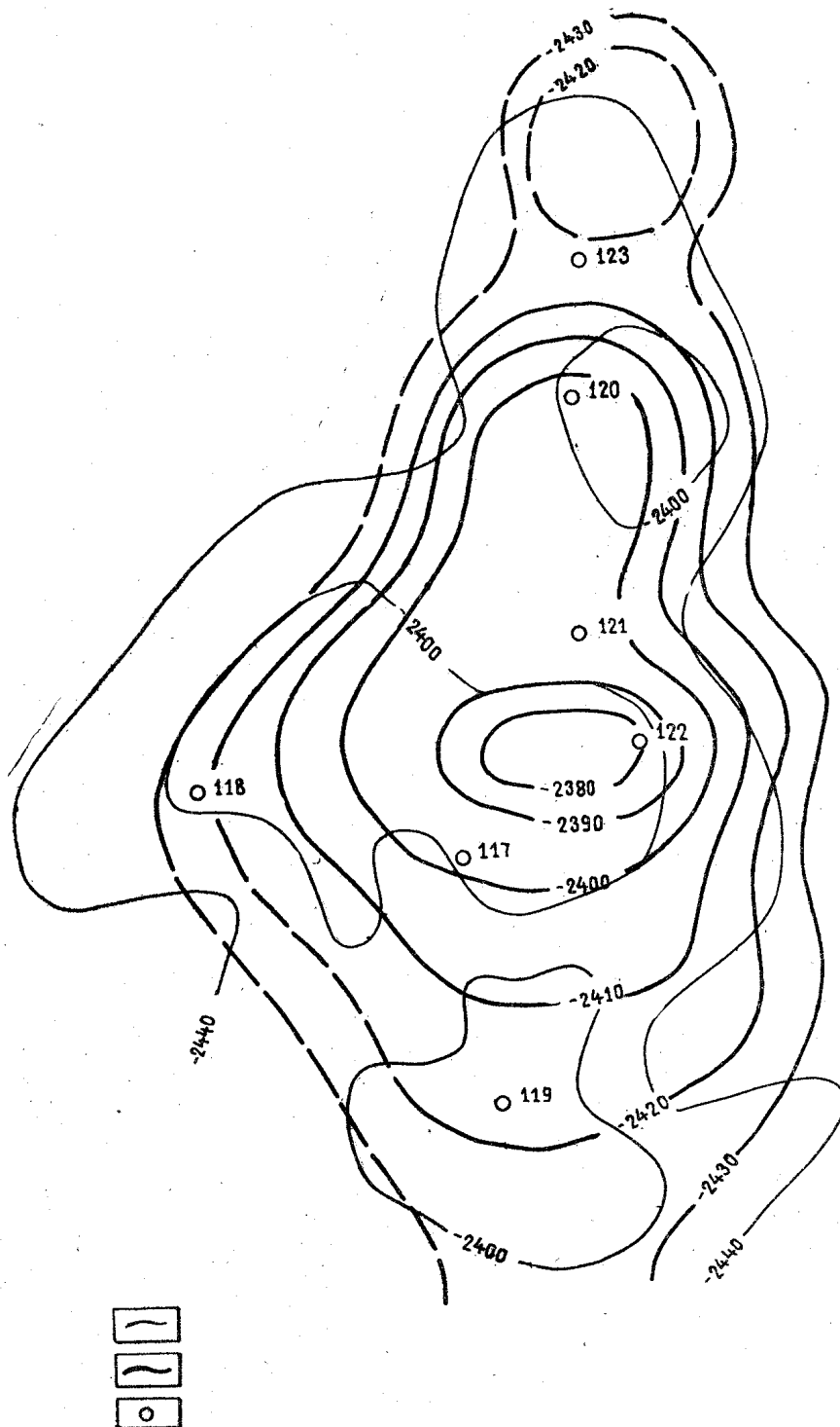
Рис. 1. Структурная карта Малореченского месторождения нефти: 1 — изогипсы по отражающему горизонту II-а (подошва марьяновской свиты валанжина); 2 — изогипсы кровли продуктивного горизонта Ю-I (васюганская свита валанжина); 3 — глубокие пробуренные скважины
