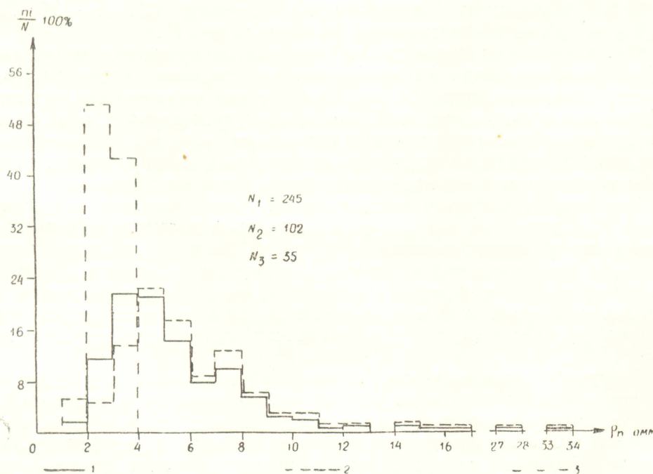
Рис. 2. Гистограмма распределения удельного электрического сопротивления \rho_{пл} песчаных и алевроитовых коллекторов горизонта А-1 (вартовская свита) Советского месторождения нефти: 1 — водонасыщенные и нефтенасыщенные пласты, 2 — нефтенасыщенные пласты по данным испытания, 3 — водонасыщенные пласты по данным испытания.
