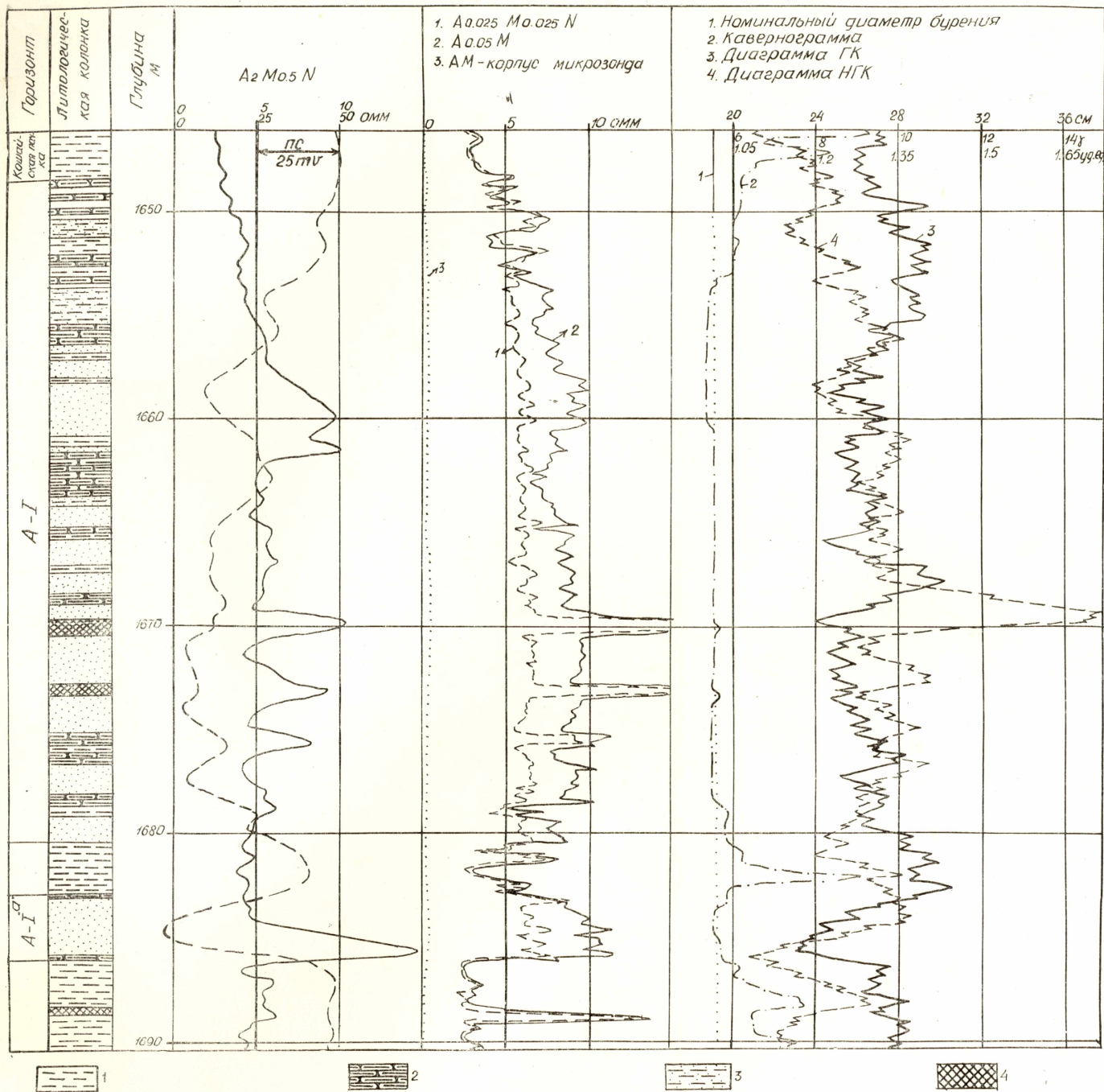
Рис. 1. Геолого-геофизический разрез горизонта A-I (вартовская свита) по скважине № 59 Советского месторождения нефти: 1—глины, 2—алевролиты, 3—глинистые песчаники, 4—плотные песчаники и алевролиты.
