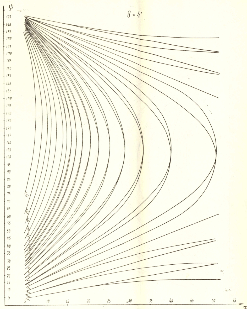
Рис. 4. Номограммы для угла скоса \delta = 4^\circ .
