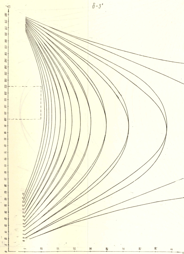
Рис. 3. Номограммы для угла скоса \delta = 3^\circ .
