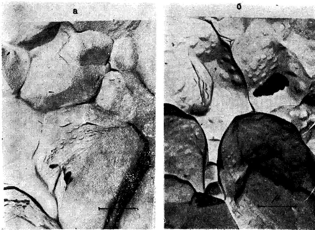
Рис. 2. Внутренние структуры в кварце с нечетко выраженной зернистой текстурой: а) кварц с структурой, обусловленной индивидами дипирамидальной формы; б) индивиды с ограничениями призмы и пирамиды
