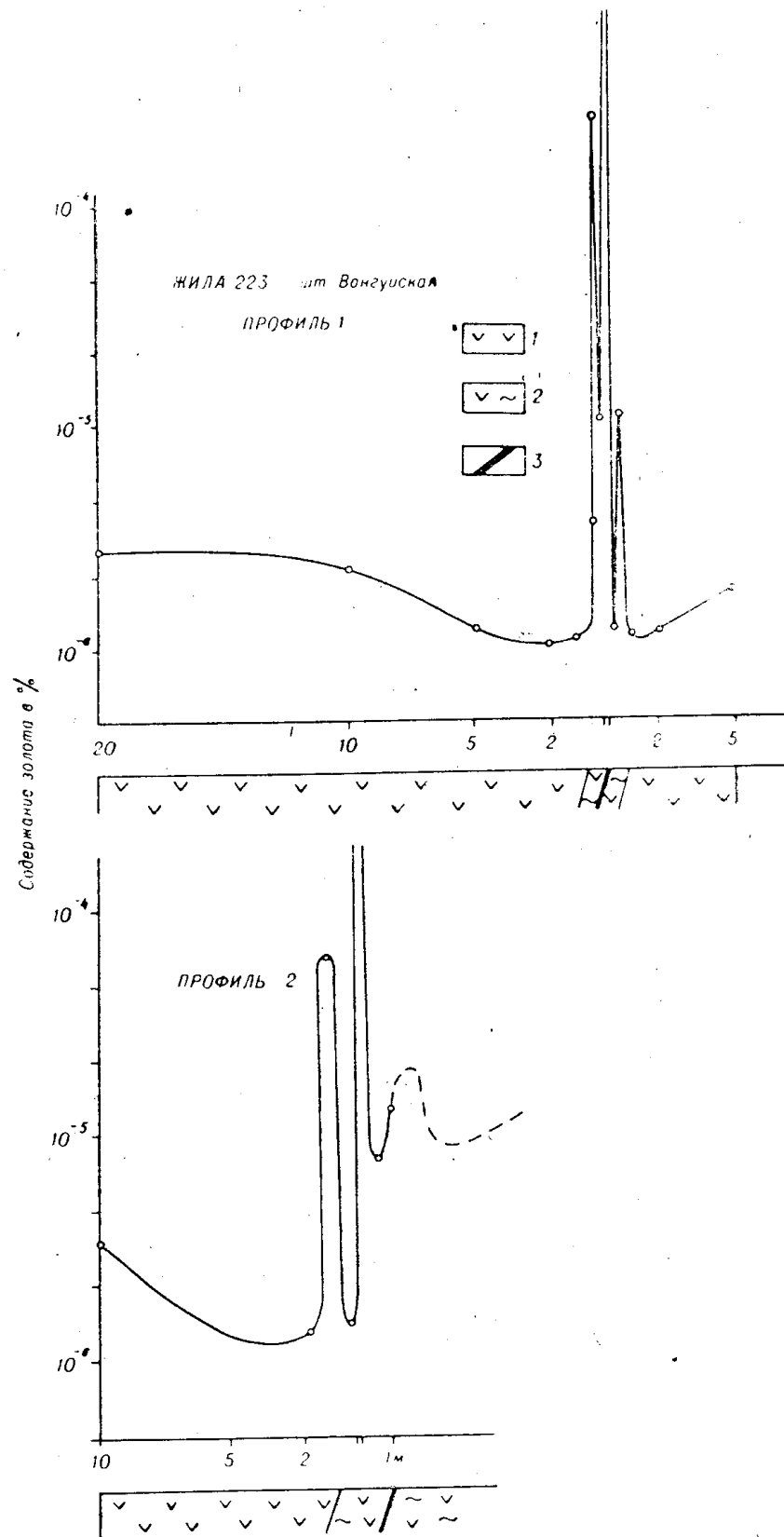
Рис. 1. Первичные ореолы золота в габбро. Дарасунское месторождение 1. Габбро. 2. Околожильно измененное габбро. 3. Золотоносная жила
