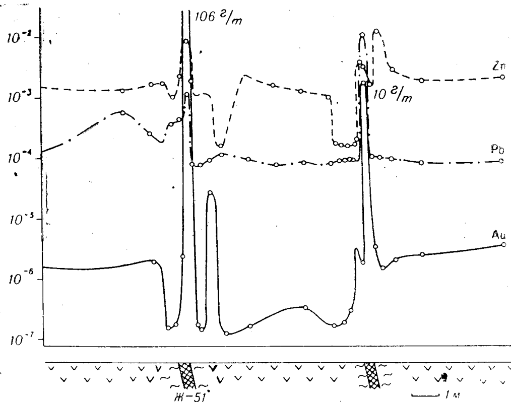
Рис. 4. Распределение золота, свинца и цинка в первичных ореолах Бериккульского месторождения
