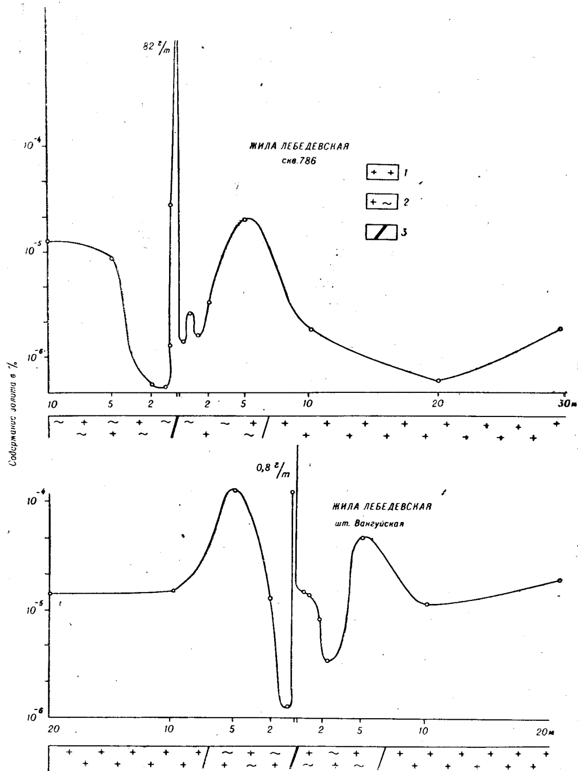
Рис. 2. Первичные ореолы золота в гранодиоритах. Дарасунское месторождение
