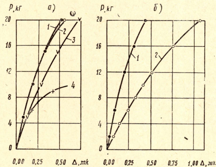
Рис. 3. а) Упругие предварительные смещения для образцов с чистотой обработки: 1/ \nabla 5 , 2/ \nabla 9 , 3/ \nabla 4 , 4/ \nabla 9 в контакте с образцом, имеющим обработку поверхности 8 класса чистоты. Коэффициенты трения соответствующих пар равны: 1/0,63, 2/0,47, 3/0,6, 4/0,2. Сталь 3, N=45 кг
