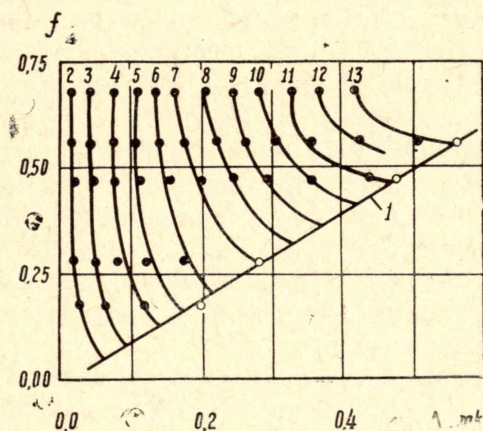
Рис. 2. Экспериментальные графики взаимосвязи предварительного смещения и коэффициент трения покоя для сил сдвига, имеющих соответственно следующие значения в кг: 1/ fN , 2/24, 3/22, 4/20, 5/18, 6/16, 7/14, 8/12, 9/10, 10/8, 11/6, 12/4, 13/2. Сталь 3, N=45 кг, чистота обработки поверхности \nabla 8 класса
