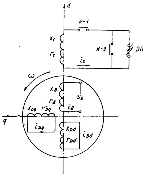
Рис. 1. Схема работы генератора на дуговой промежуток
