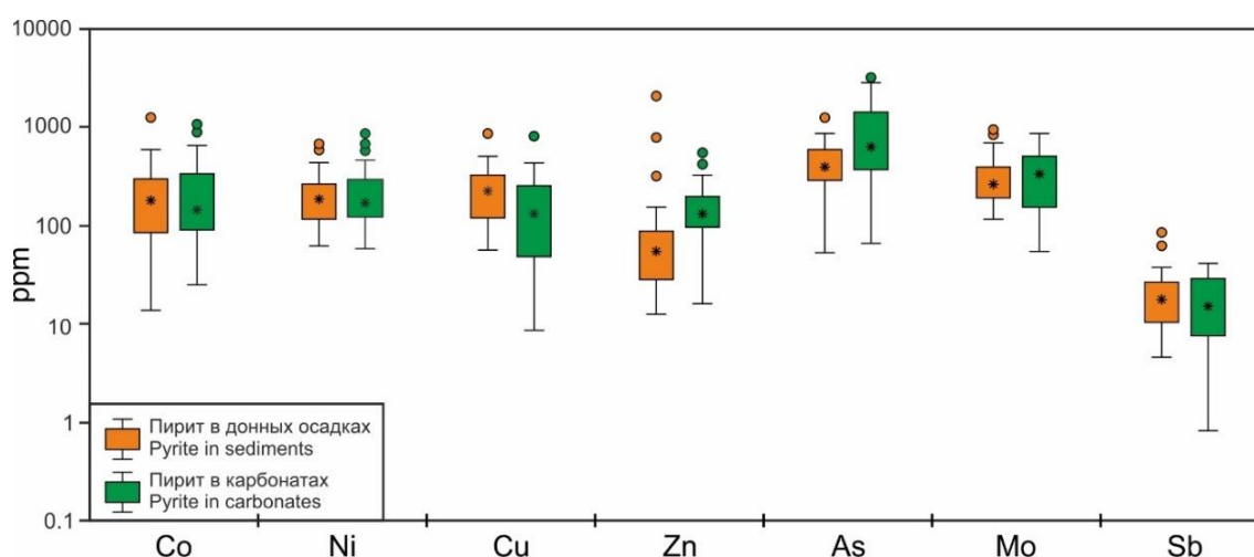
Рис. 6. Микроэлементный состав пирита в изученных образцах донных осадков и карбонатных корок по данным ЛА-ИСП-МС. Звездочки внутри ящичков обозначают медиану, границы ящичков соответствуют 25-му и 75-му перцентилям, «усы» показывают диапазон значений без выбросов, а точки отражают выбросы
