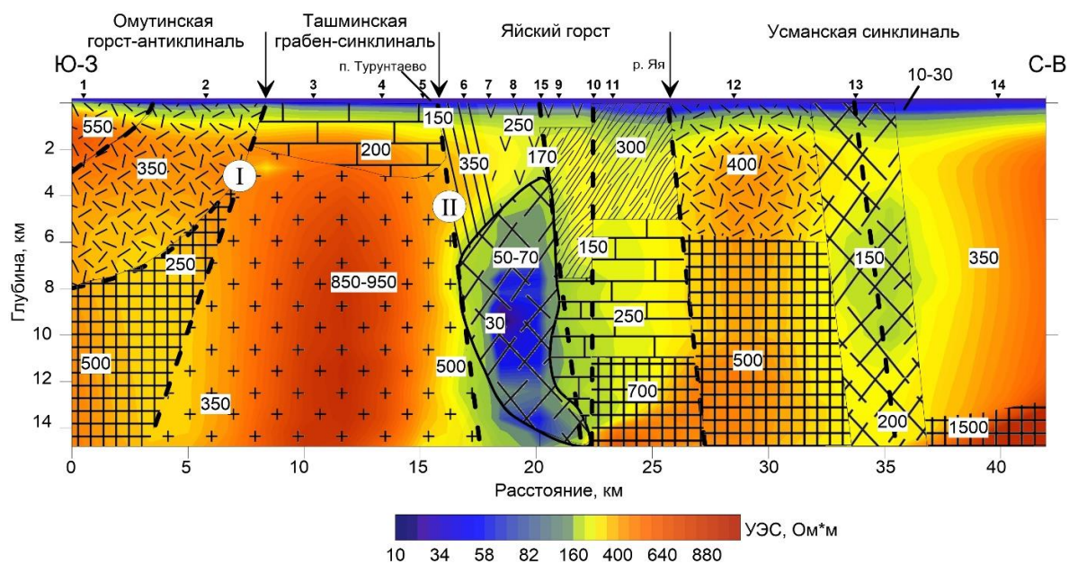
Рис. 3. Разрез УЭС по результатам МТЗ с элементами интерпретации: 1 – гранитоидный комплекс; 2 – додевонские (каледонские) структурные комплексы; 3 – известняки, песчаники, алевролиты; 4 – субвулканические образования: шток и дайкообразные тела; 5 – лавы, туфы, базальты, туфопесчаники; 6 – андезиты, базальты, туфы; 7 – зона флюидно-магматической переработки с повышенной трещиноватостью пород; 8 – хлорит-серицитовые сланцы; 9 – оси смещения основных разломов; I – Томский шарьяж; II – Кузнецко-Алатаусский разлом
