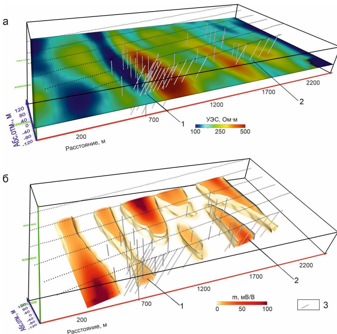
Рис. 6. Распределение УЭС (а) и поляризуемости (б) на уровне рудовмещающей толщи по результатам 3D-инверсии; цифрами отмечены участки: 1 – Центральный, 2 – Восточный; 3 – скважины
