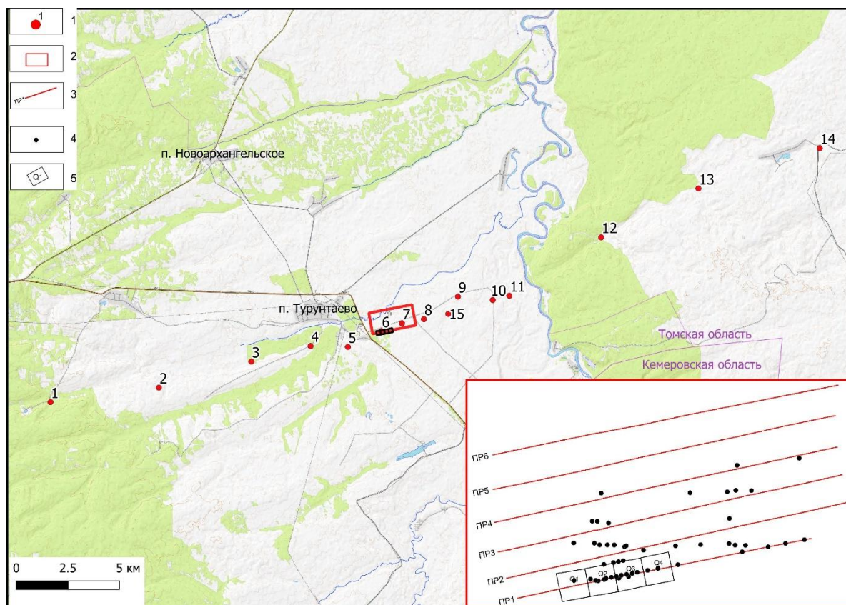
Рис. 2. Схема полевых исследований: 1 – пункты МТЗ и их номер; 2 – положение участка работ ЭТ-ВП; 3 – профили ЭТ-ВП и их номер; 4 – положение скважин; 5 – генераторные петли метода зондирования становления поля
