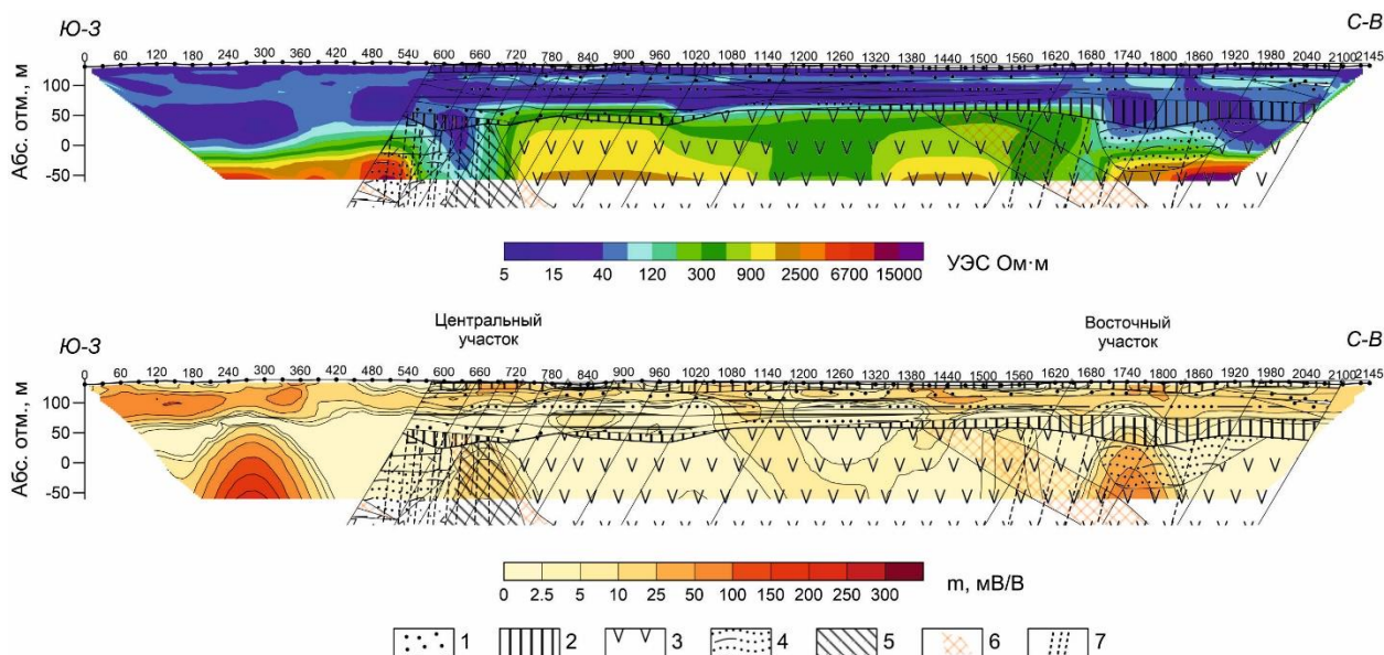
Рис. 5. Разрез УЭС профиля № 1 вдоль буровой линии (а), поляризуемости (б) с элементами интерпретации по результатам 2D-инверсии: 1 – песок; 2 – глина; 3 – плагиоклазовые порфириты; 4 – туфопесчаники и туфогравелиты; 5 – хлорит-серицитовые метасоматиты; 6 – кварц-карбонатные метасоматиты переходной зоны; 7 – разломы
