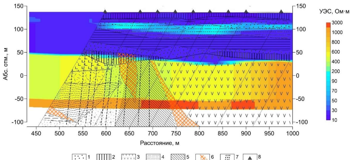
Рис. 4. Разрез УЭС по результатам зондирования становлением поля (ЗС) с элементами интерпретации: 1 – песок; 2 – глина; 3 – плагиоклазовые порфиристы; 4 – туфопесчаники и туфогравелиты; 5 – хлорит-серицитовые метасоматиты; 6 – кварц-карбонатные метасоматиты переходной зоны; 7 – разломы; 8 – положение скважины
