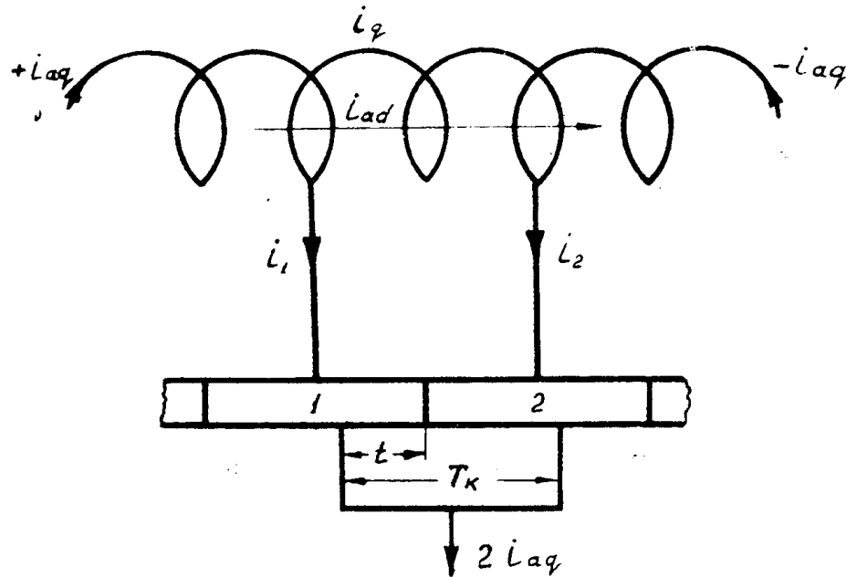
Рис. 7. Схема коммутируемого контура поперечной цепи.
