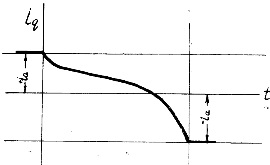
Рис. 1. Кривая тока поперечной цепи при b_{ин} = b_{к} .
