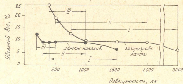
Рис. 1. Удельный вес общего освещения в системе комбинированного
