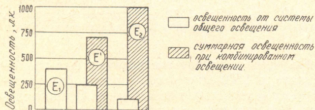
Рис. 2. Соотношение освещенности для трех систем освещения
