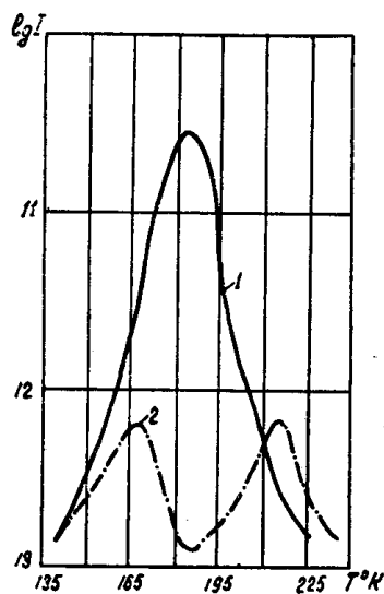
Рис. 3. Зависимость тока деполяризации от температуры для кристаллов \text{KBr} + 0,02 \text{ M\% KOH} (1) и \text{KBr} + 0,01 \text{ M\% PbCl}_2 (2)
