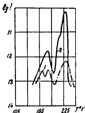
Рис. 1. Зависимость тока деполаризации от температуры для кристаллов KCl (1) и KCl + 0,25 M% SrCl 2
