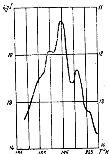
Рис. 2. Зависимость тока деполаризации от температуры для кристаллов KBr
