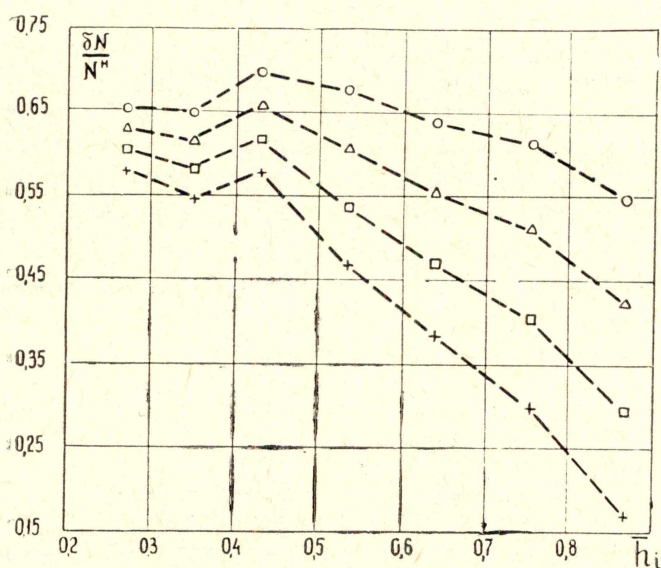
Рис. 3. Зависимость относительных приростов мощности в процентах от величины относительного использования теплоперепада вытесняемого отбора пара при разных \eta_{oi} турбины АФ: + — \eta_{oi} = 0 ; □ — \eta_{oi} = 0,3 ; Δ — \eta_{oi} = 0,6 ; ○ — \eta_{oi} = 0,9
