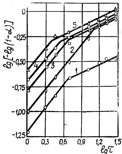
Рис. 2. Зависимость \lg[-\lg(1-a)] от \lg \tau для процесса сернокислотного разложения фтористого магния при различных температурах: 1 — 100° С, 2 — 150° С, 3 — 200° С, 4 — 230° С, 5 — 250° С
