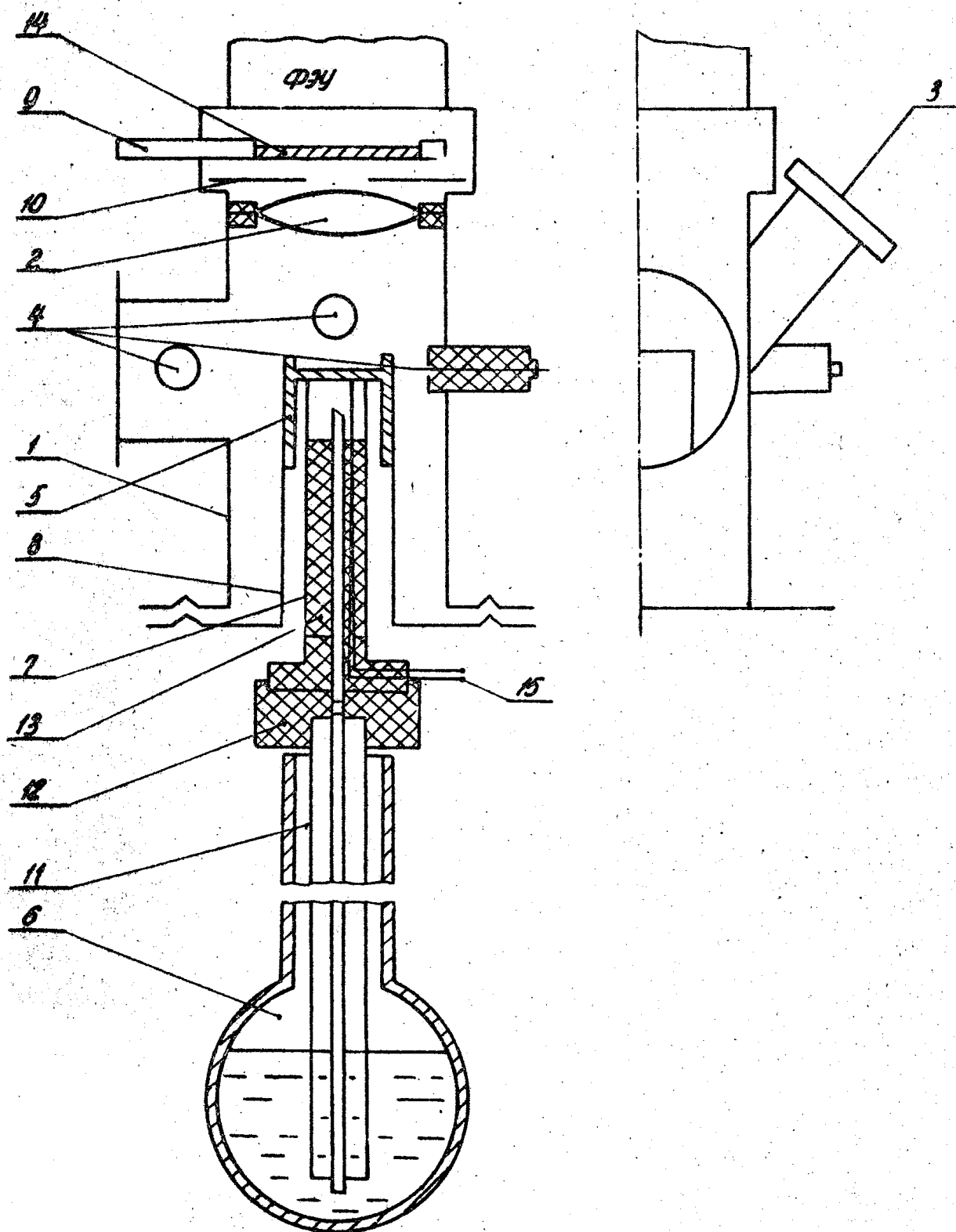
Рис. I I3-изоляция, I4-светофильтр, I5-термопара.
