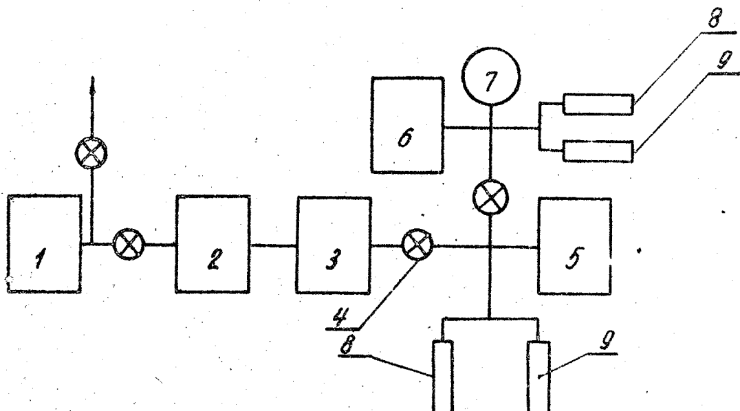
Рис.3. 1-насос форвакуумный ВН-46I, 2-насос пароструйный НВО-40, 3-ловушка азотная, 4-клапаны, 5-ячейка, 6-титановый насос, 7-датчик масс-спектрометра РМО-4, 8-датчик давления ЛМ-2, 9-датчик давления ЛТ-2.
